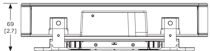
Vista trasera
