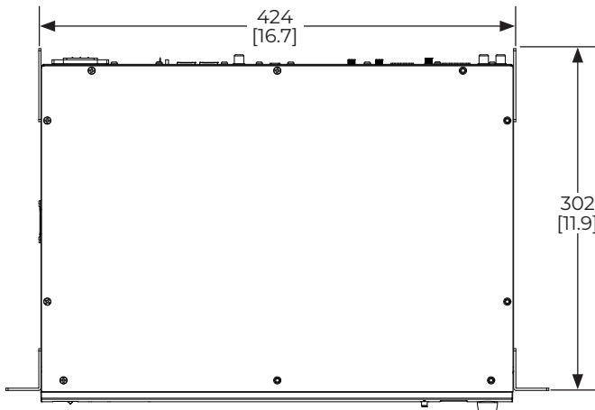
Vista superior 8
