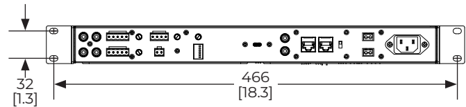
Vista trasera
