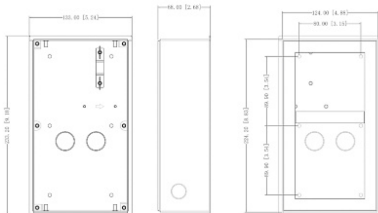
Dimensiones con 3 elementos combinados - parte frontal:
