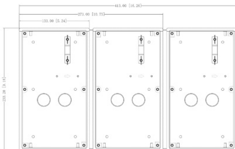
Dimensiones con 3 elementos combinados - parte trasera:
