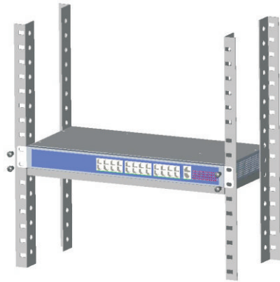
Figura 2-2 Instale el interruptor en el bastidor
