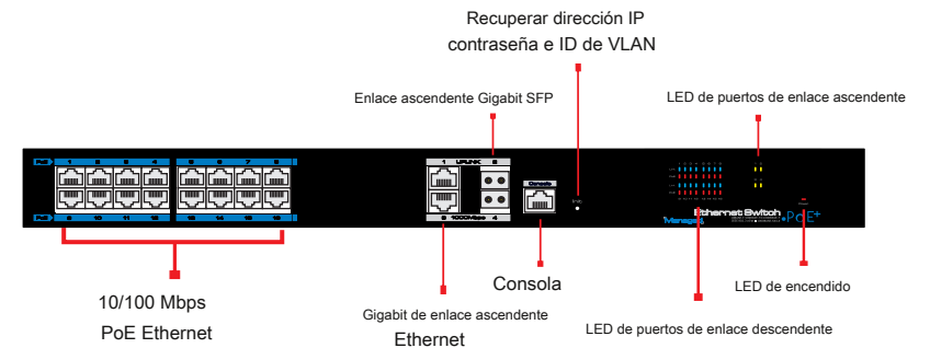
Panel frontal del switch PoE administrable de 16 puertos
