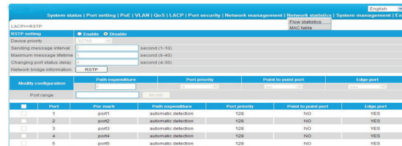
Figura 4-6 RSTP
