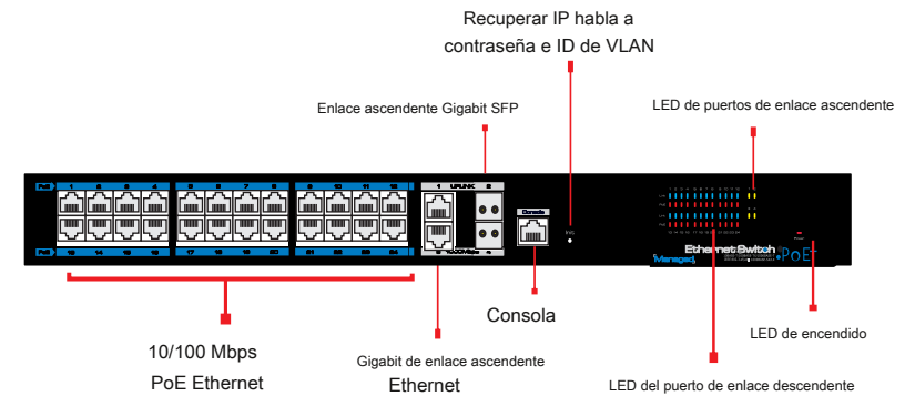
Panel frontal del switch POE administrable de 16 puertos
