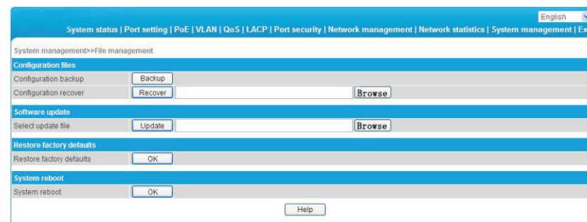
Figura 4-18 Gestión de documentos
