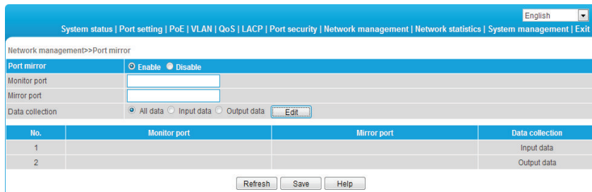
Figura 4-11 Puerto espejo
