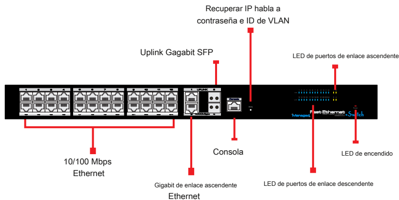
Panel frontal del switch POE administrable de 24 puertos
