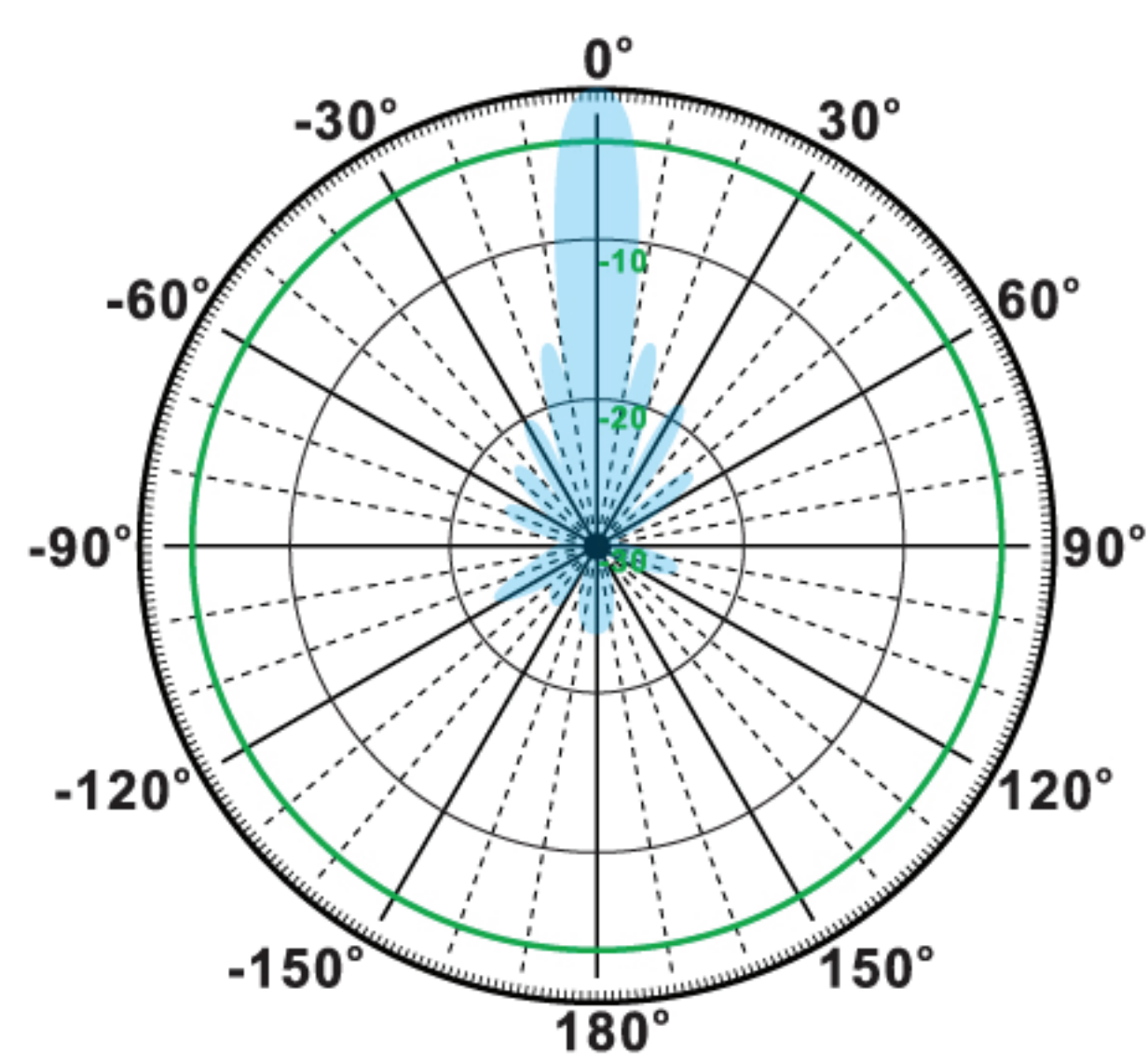
H-Plane
