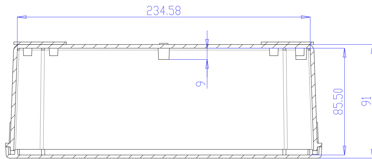
SECCIÓN A-A
