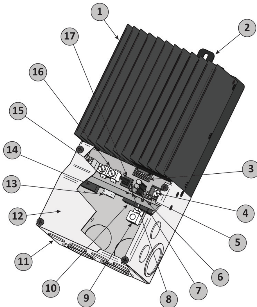
característica.Figura 2-1. TriStar MPPT características
