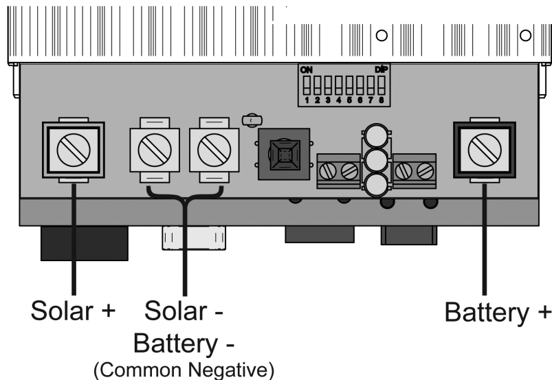
Figura 3-7. Ubicación de los terminales eléctricos
