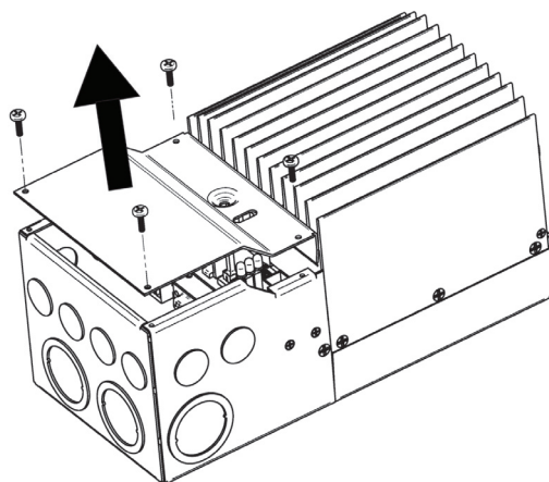
Figura 3-1. Quite la tapa de la caja de conexiones.
