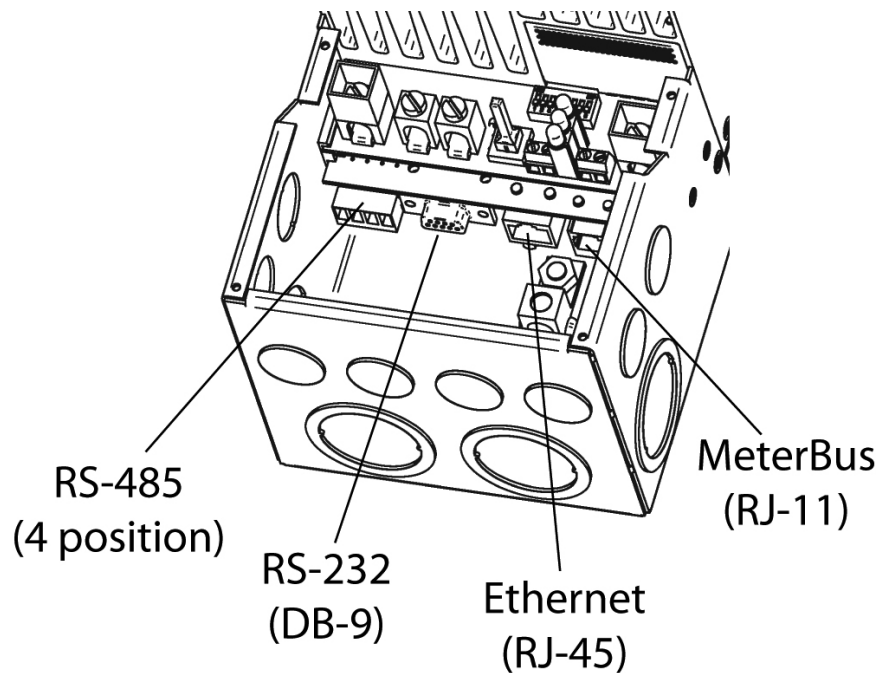
Figura 3-5. Ubicación de conectores de red del TriStar MPPT
