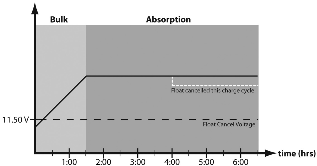
Figura 4-5. Perfil de carga con cancelación de estado flotante
