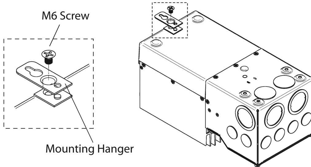
Figura 3-2. Colocación del soporte de montaje
