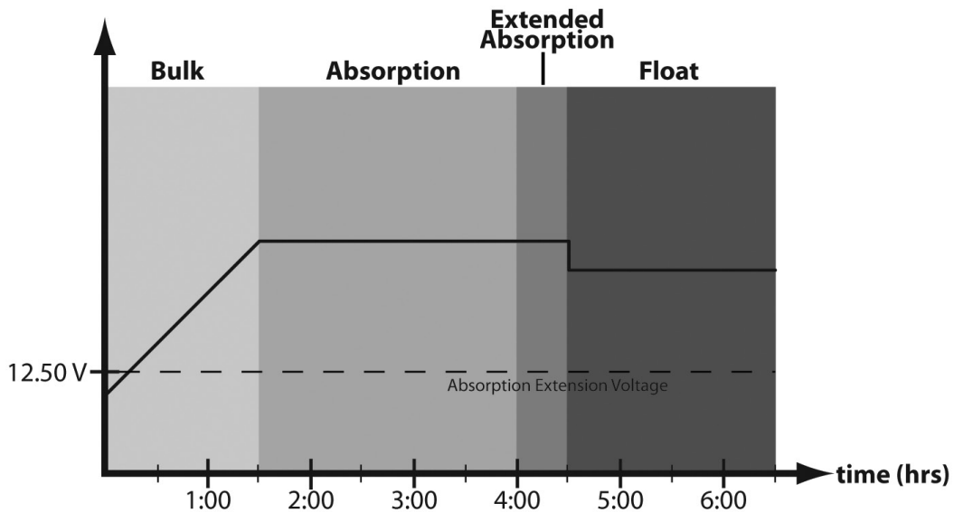
Figura 4-3. Perfil de carga con extensión de absorción.
