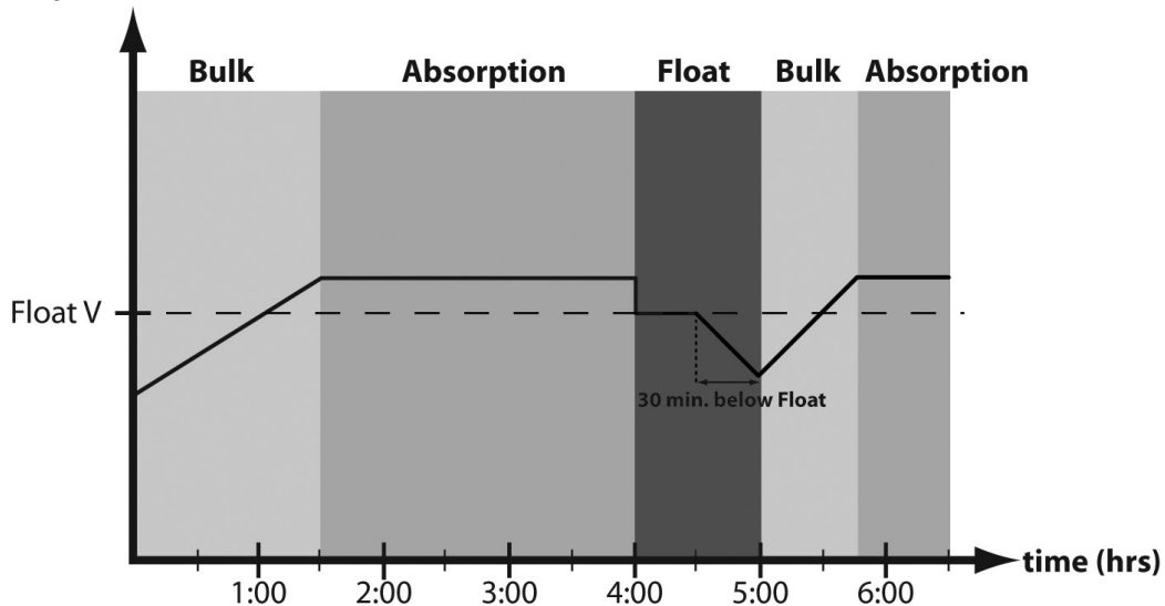
Figura 4-4. Perfil de carga con tiempo de carga flotante
