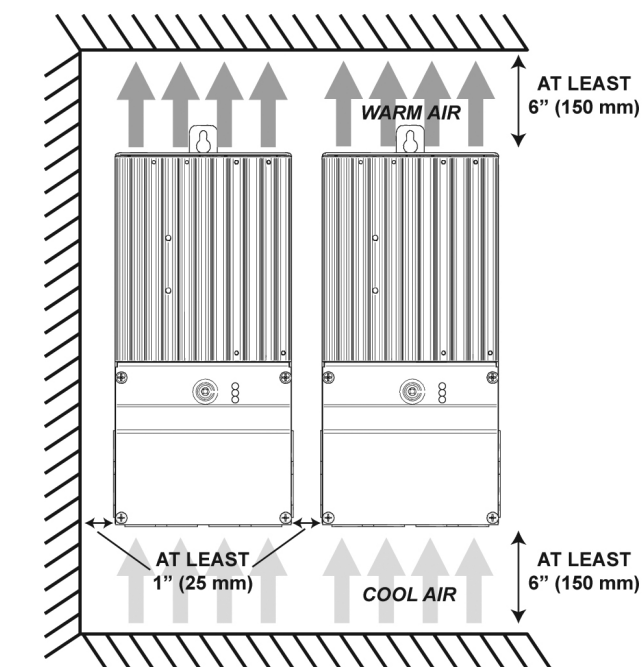
Figura 3-3. Distancias de montaje para que circule aire.
