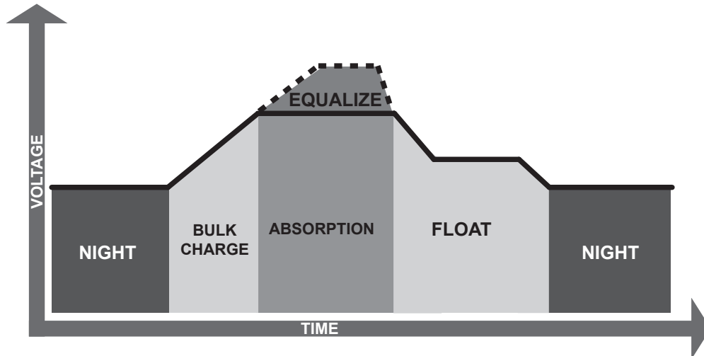
Figura 4-2. Algoritmo de carga del TriStar MPPT
