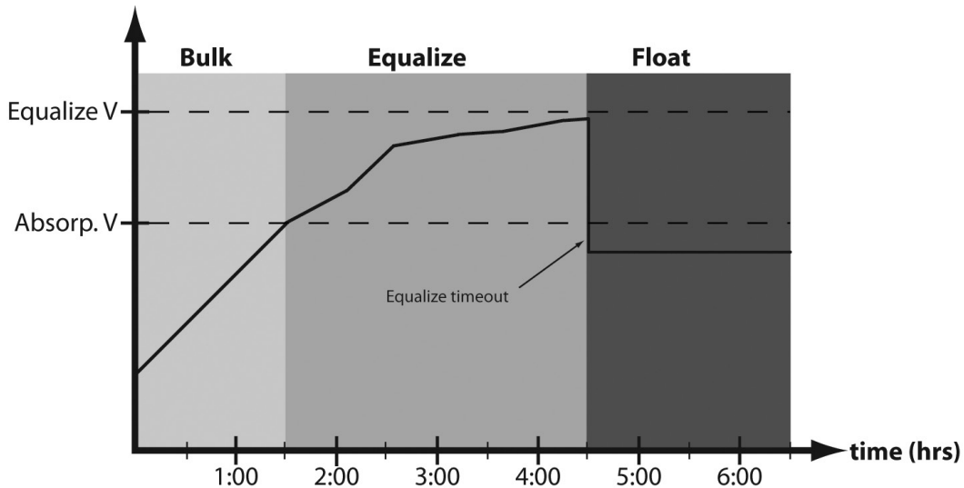
Figura 4-6. Perfil de carga con tiempo de ecualización
