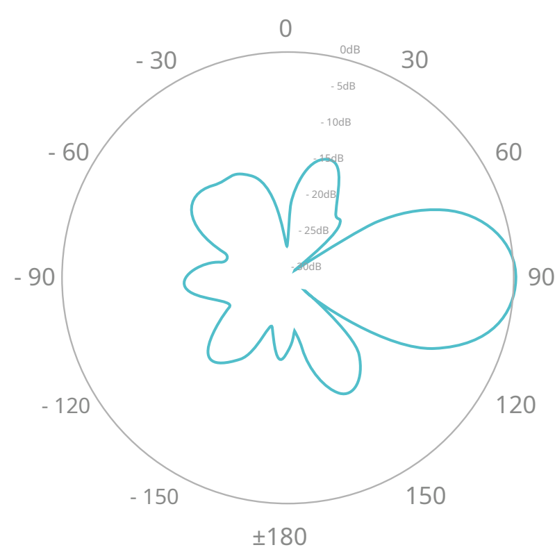
Elevación Horizontal
