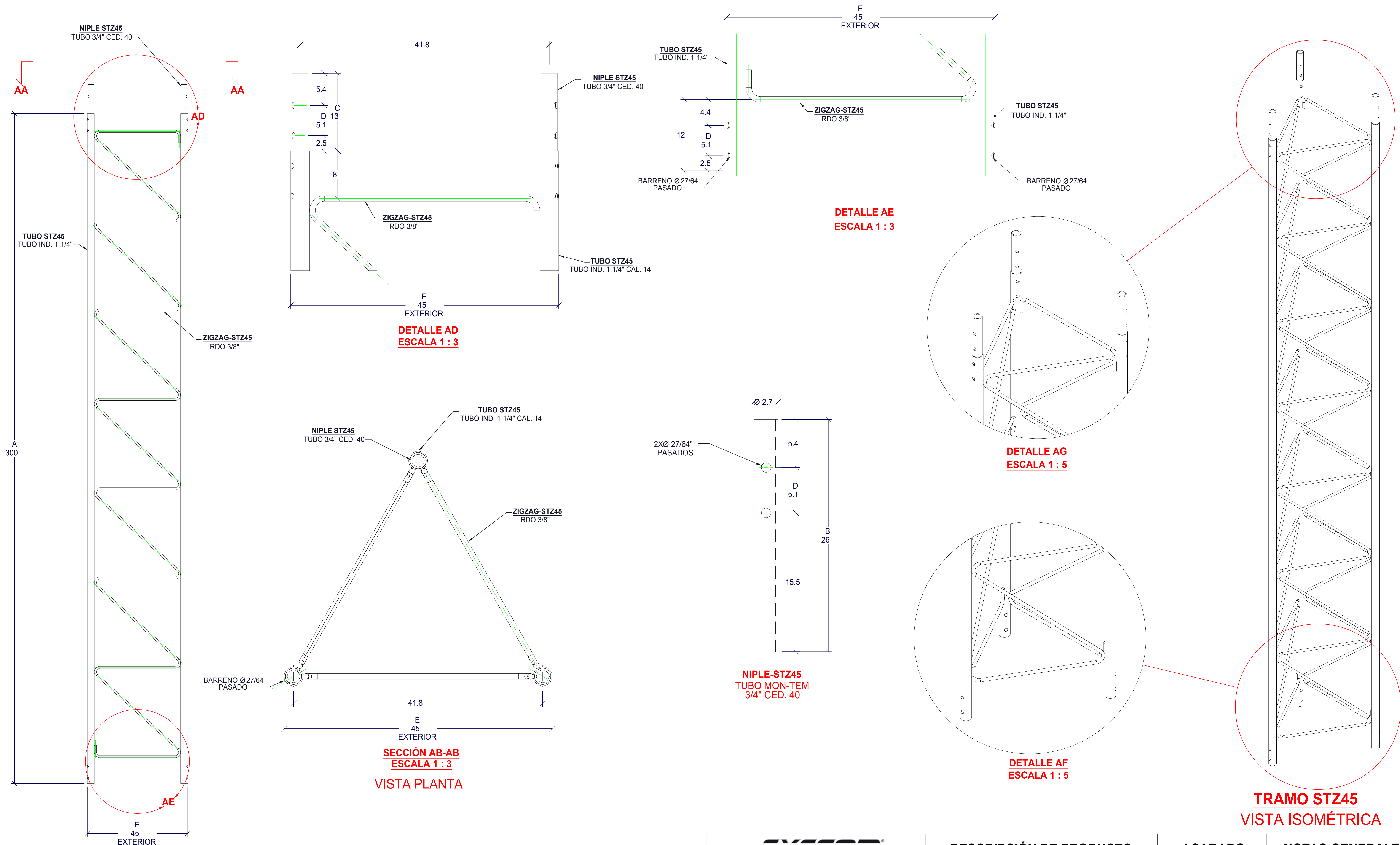
TRAMO MODELO STZ45 VISTA FRONTAL
