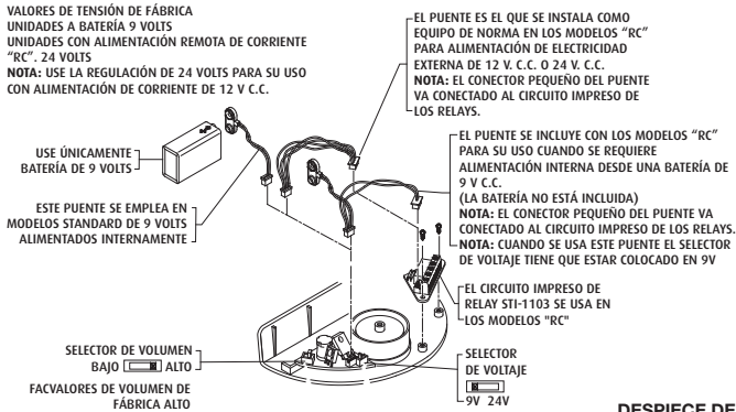
DESPIECE DE LA PARTE ELECTRÓNICA FIG. 6
