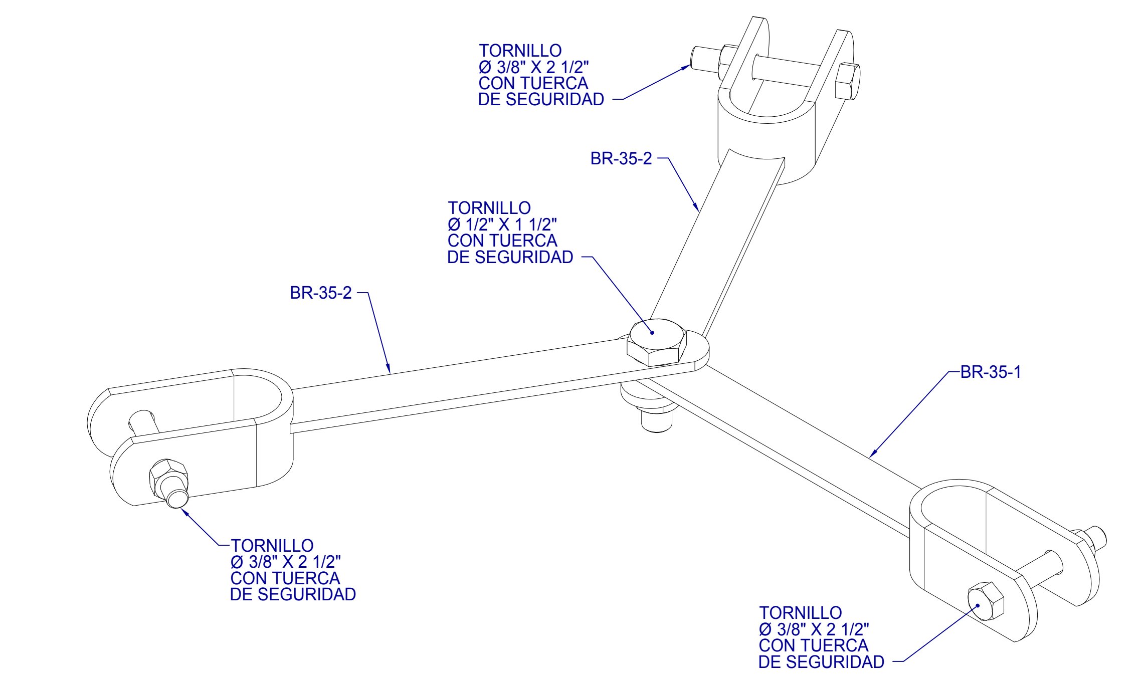
VISTA ISOMETRICA ENSAMBLAJE BRIDA 35
