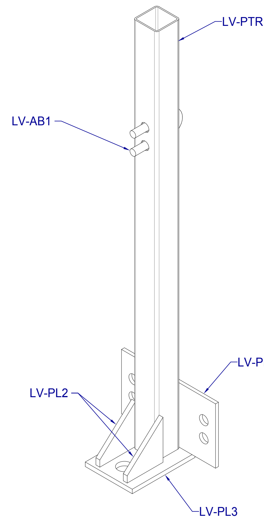
VISTA ISOMÉTRICA HERRAJE SUJECIÓN DE LÍNEA DE VIDA
