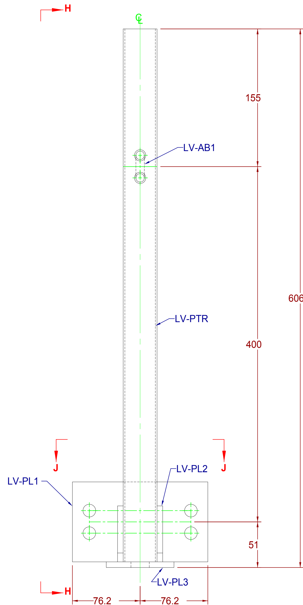
VISTA ELEVACIÓN HERRAJE SUJECIÓN DE LÍNEA DE VIDA
