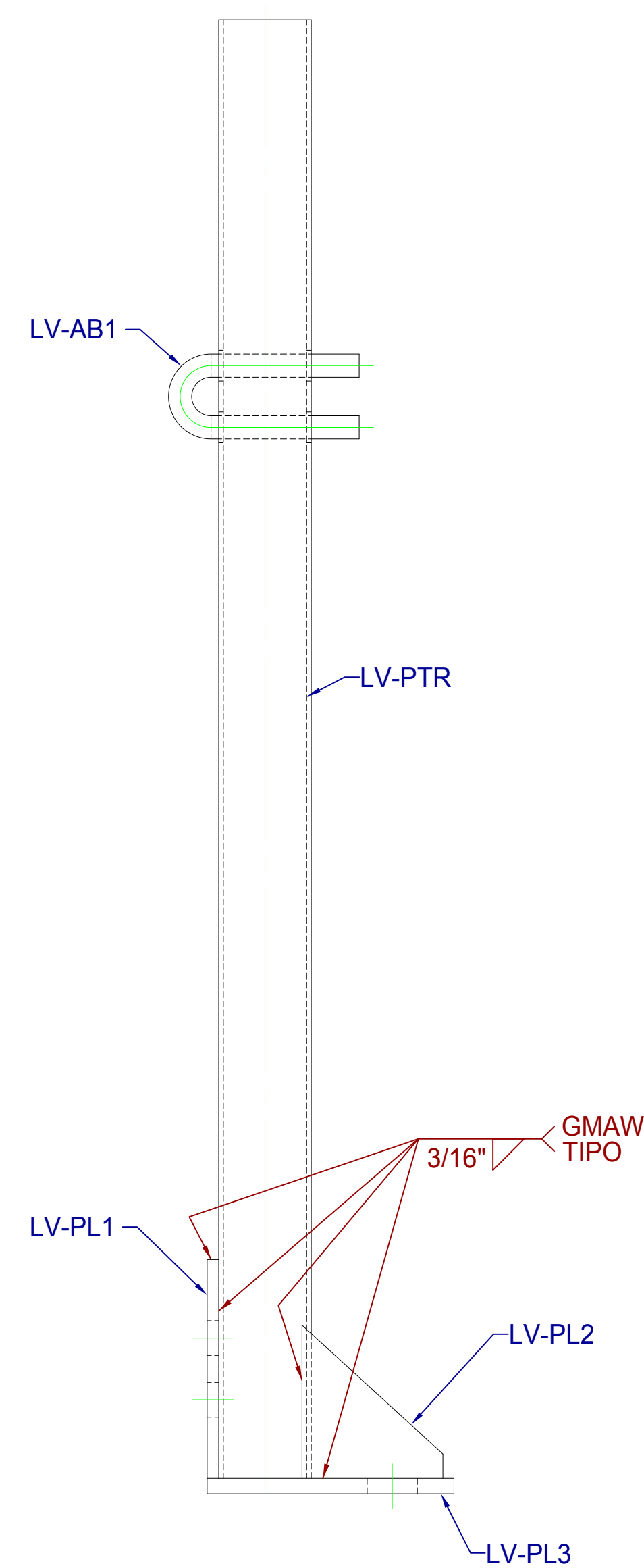
SECCIÓN H-H ESCALA 1:2
