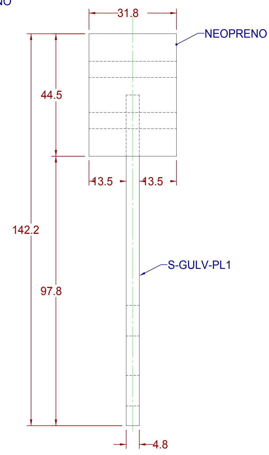
SECCIÓN H-H ESCALA 2 : 1.5
