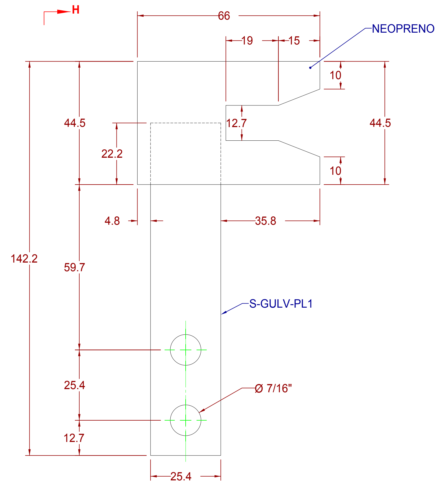
VISTA ELEVACIÓN GUÍA PARA LÍNEA DE VIDA S-GULV
