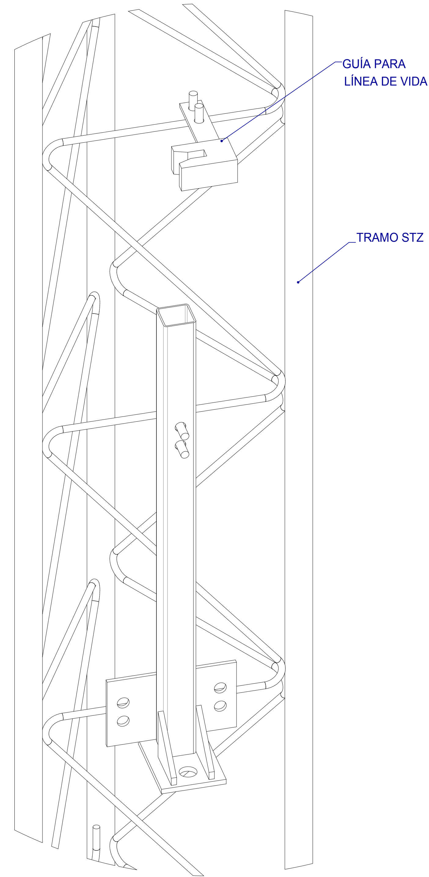
DETALLE J ESCALA 2 : 5
