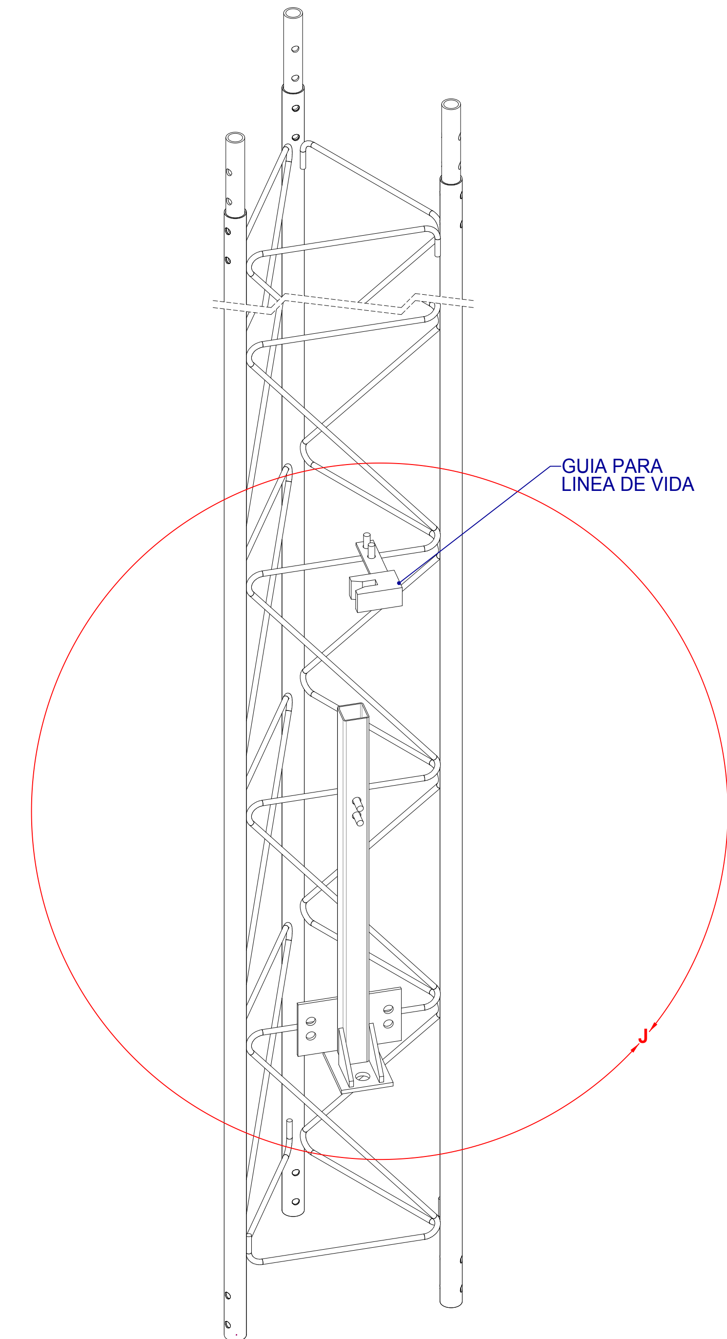
VISTA ISOMÉTRICA MONTAJE GUÍA PARA LÍNEA DE VIDA S-GULV
