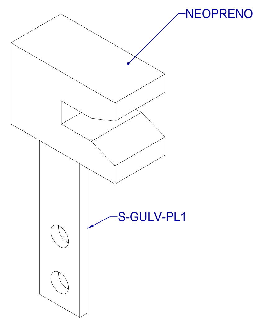
VISTA ISOMÉTRICA GUÍA PARA LÍNEA DE VIDA S-GULV
