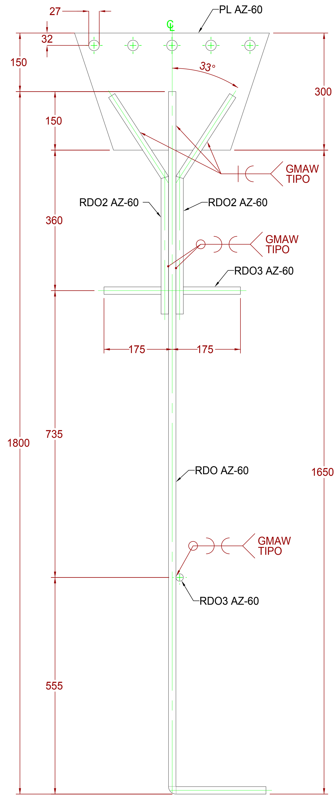
ELEVACION FRONTAL Y LATERAL ANCLA SAZ-60G
