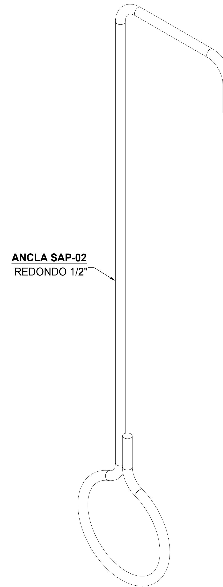
ANCLA SAP-02 VISTA ISOMETRICA
