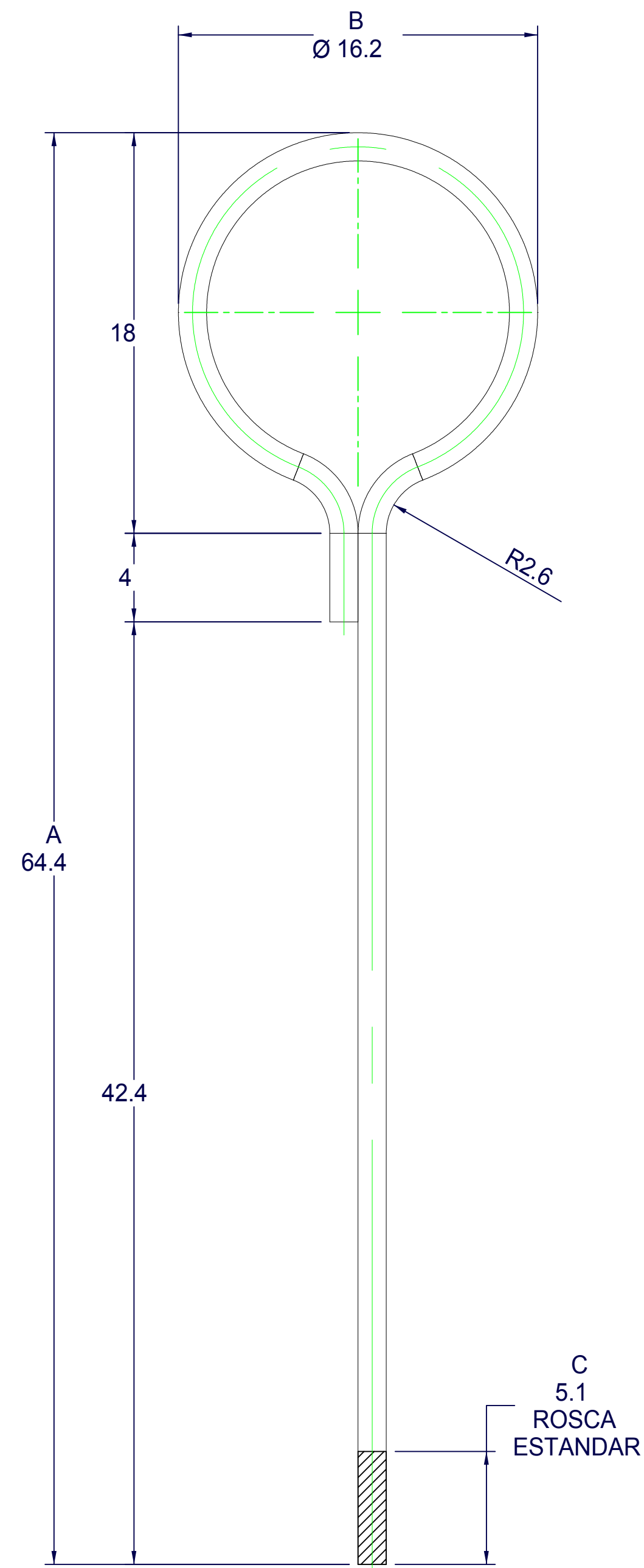
ANCLA SAP-01 (1 PZA) REDONDO LISO Ø 1/2" DESARROLLO: 995 MM
