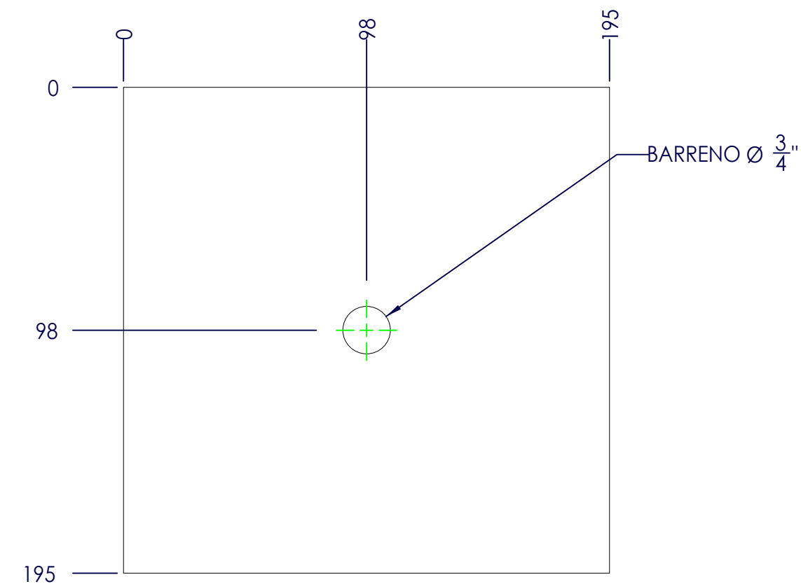
OL-PL1 (1 PZA) PLACA 1/4"
