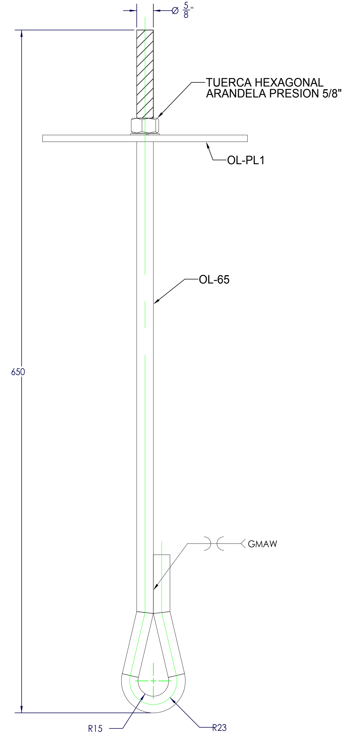
ENSAMBLE ANCLA SAP01J
