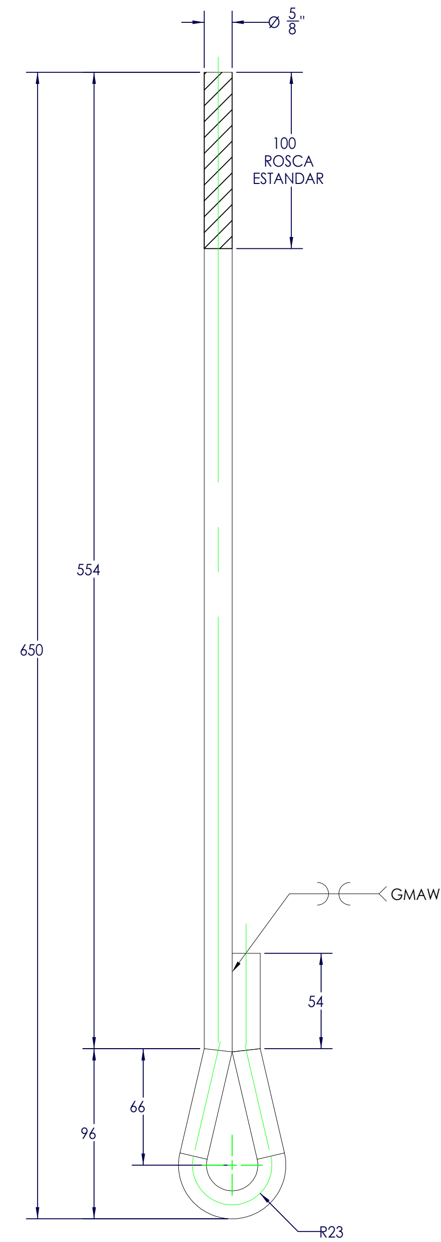
OL-65 (1 PZA) RDO. 5/8" DESARROLLO CORTE 814 mm
