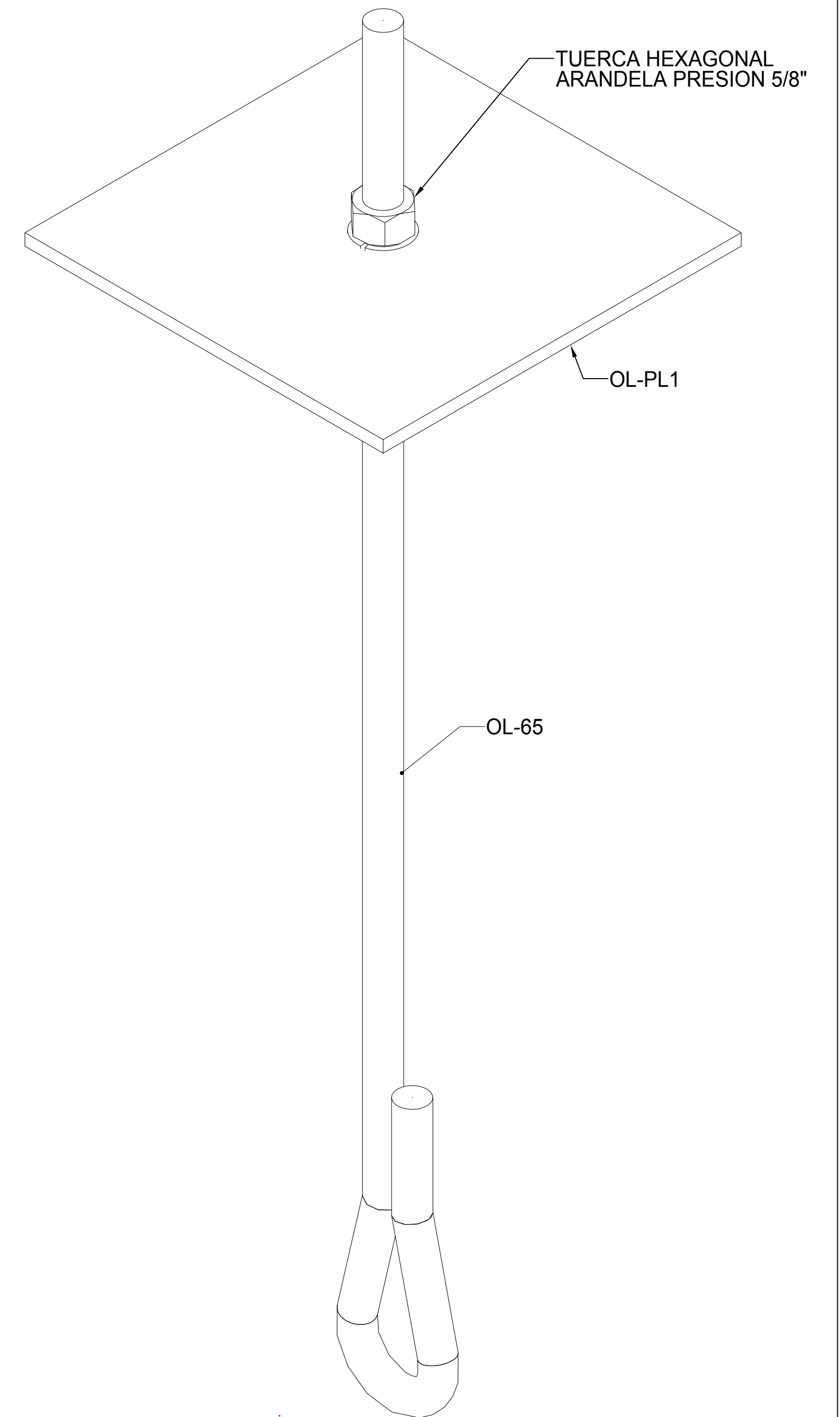
VISTA ISMETRICA ANCLA SAP01J
