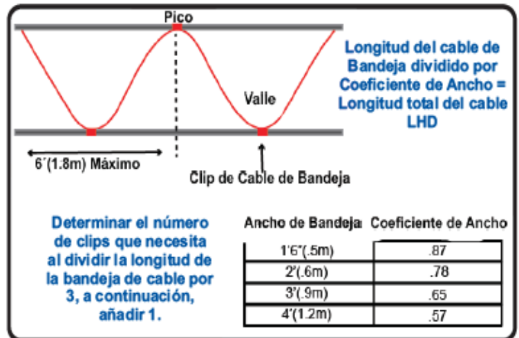
Cálculo de la onda sinusoidal de la bandeja de Cable
