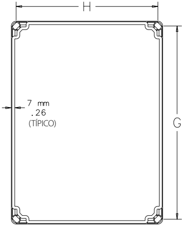
VISTA INFERIOR
