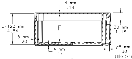
SECCIÓN C-C
