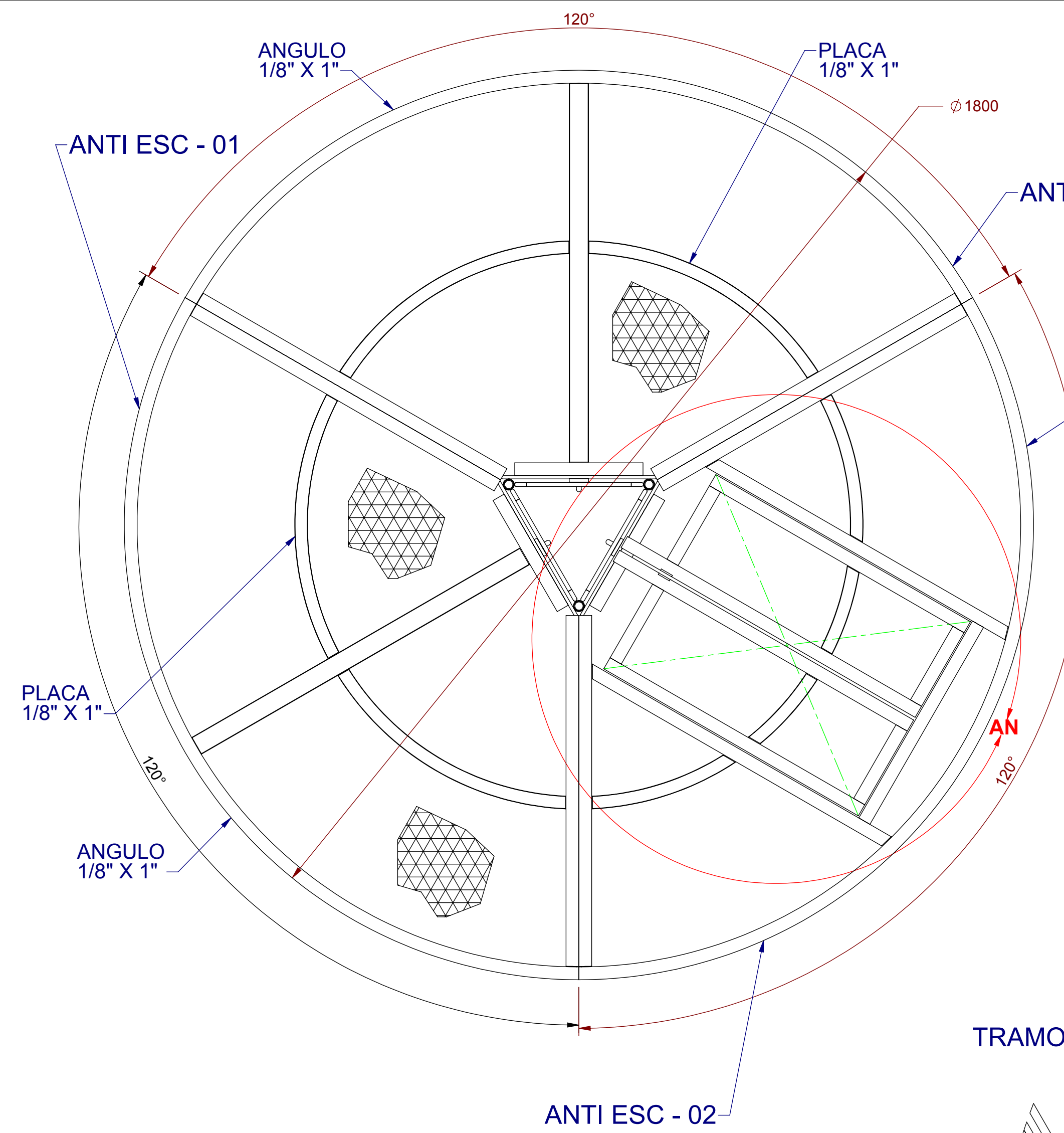
MONTAJE VISTA PLANTA SOMBRILLA ANTI ESCALA SOM30
