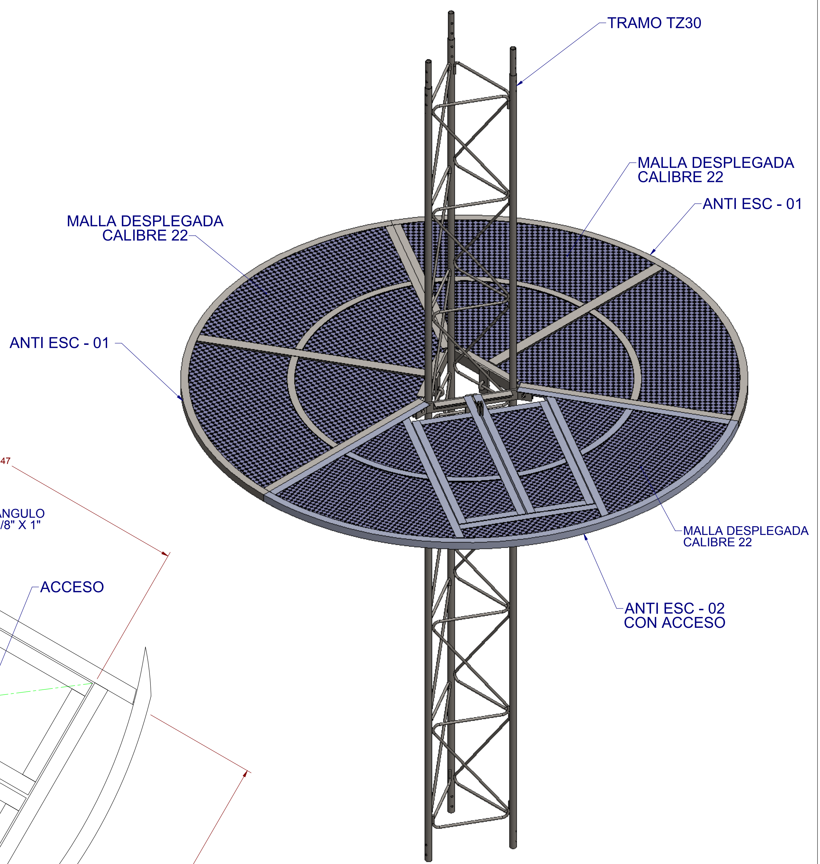
MONTAJE SOMBRILLA ANTI ESCALA SOM30
