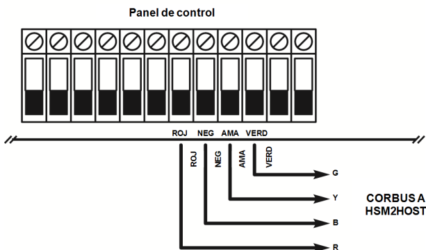
Figura 2-6 Diagrama de cableado del HSM2HOSTx
