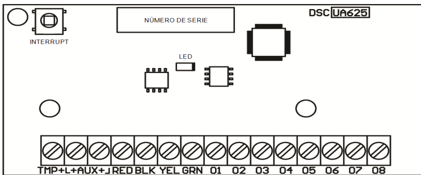
Figura 2-5 HSM2208 Expansor de salida
