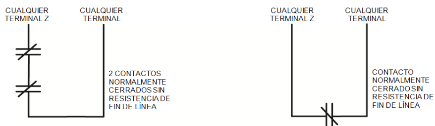
Figura 2-9 Normalmente cerrado
