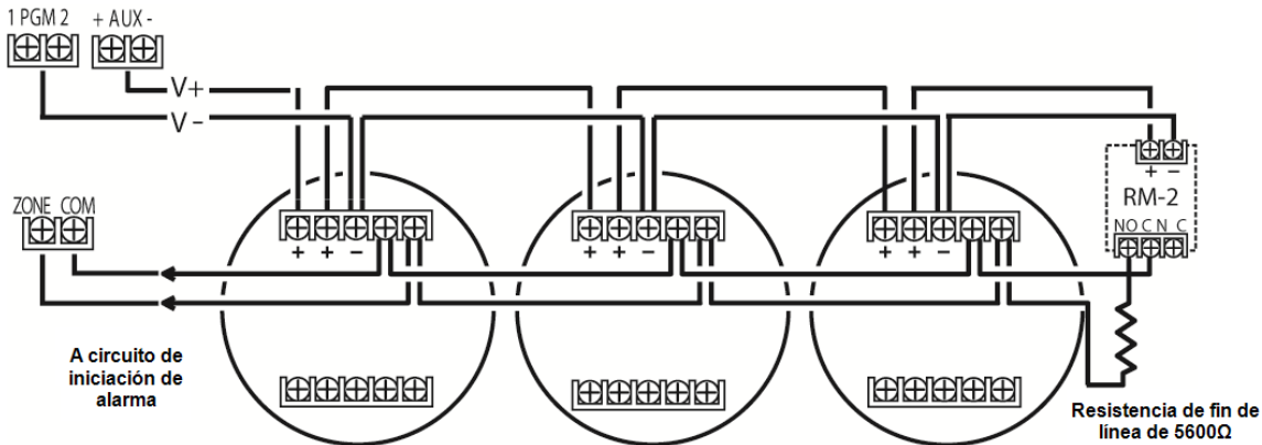
Figura 2-15 Cableado del detector de humo
