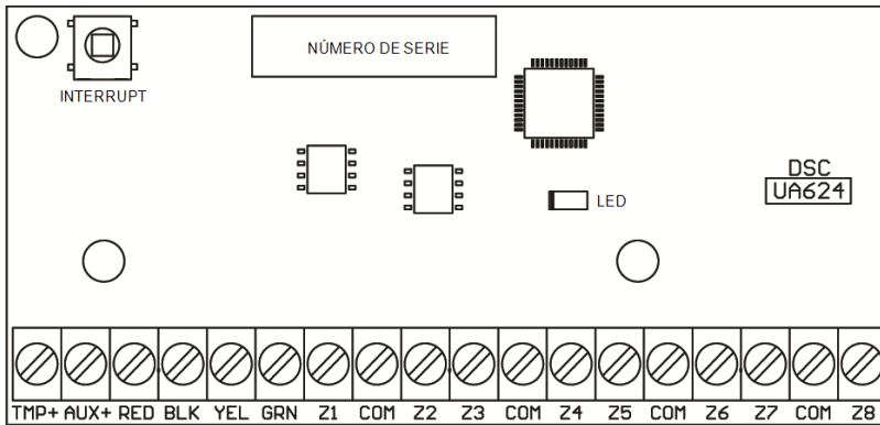
Figura 2-4 HSM2108 Expansor de zona
