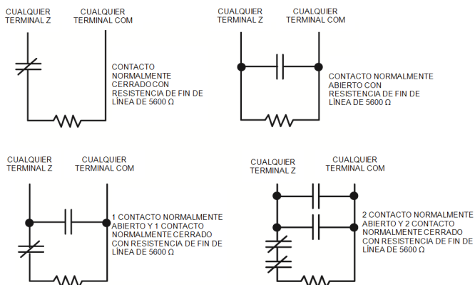
Figura 2-10 Cableado de SEOL
