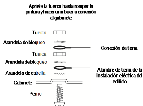
Figura 2-18 Instalación de tierra
