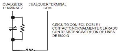
Figura 2-11 Cableado de DEOL
