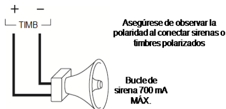
Figura 2-13 Cableado de terminales sirena
