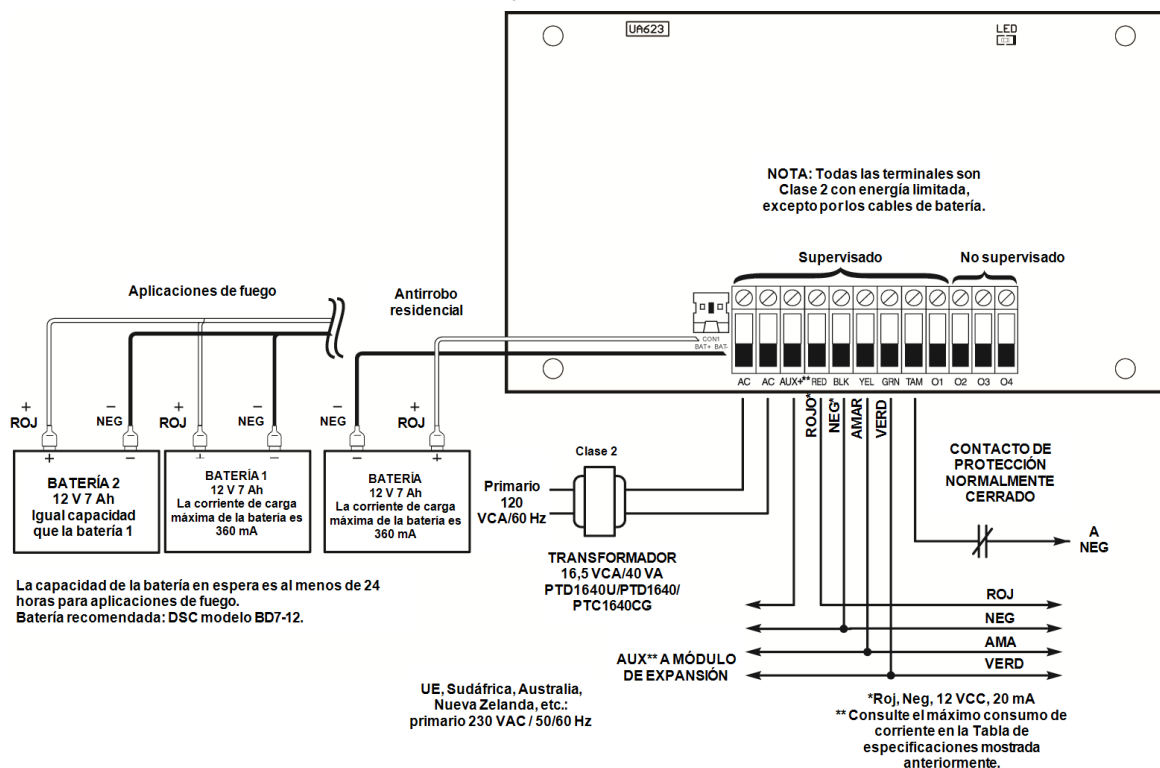
Figura 2-7 Cableado de la fuente de alimentación
