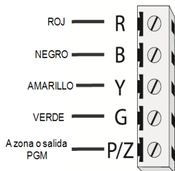
Figura 2-8 Terminales P/Z del teclado
