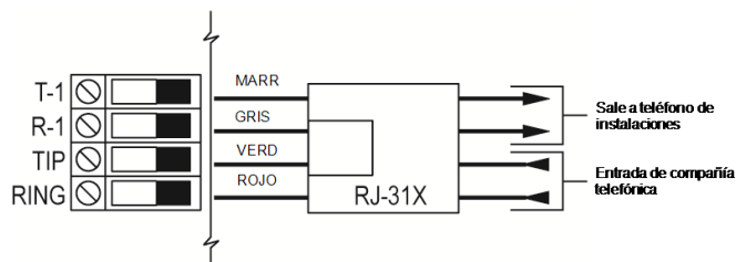
Figura 2-14 Cableado de línea telefónica
