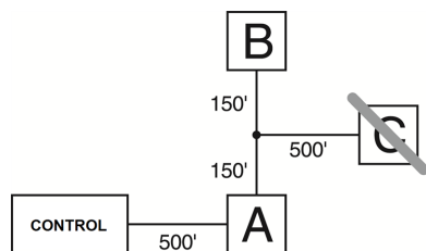
Figura 2-3 Cableado Corbus
