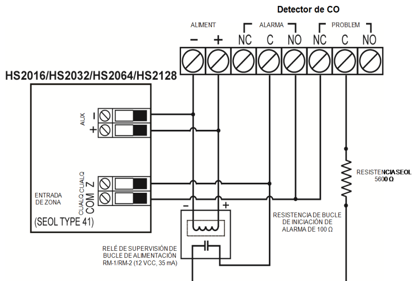
Figura 2-17 Cableado del detector de CO
