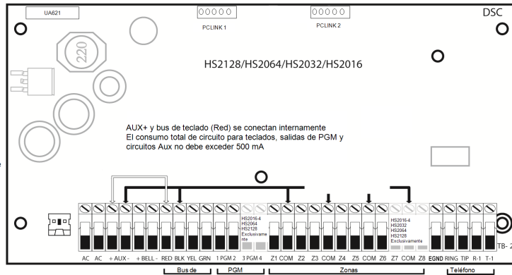
Figura 2-2 Enrutamiento de cableado (exclusivo para EN50131)
