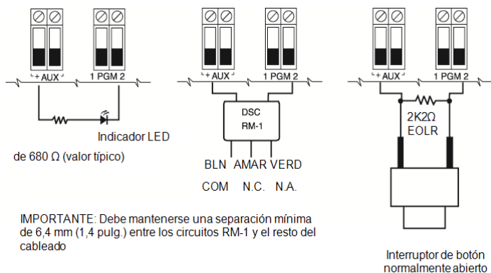
Figura 2-12 Salida LED con resistencia limitadora de corriente y salida opcional de controlador de relé.
