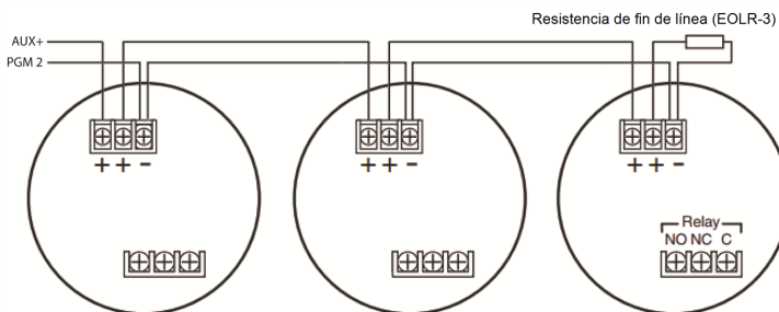
Figura 2-16 Cableado de detector de humos de dos hilos
