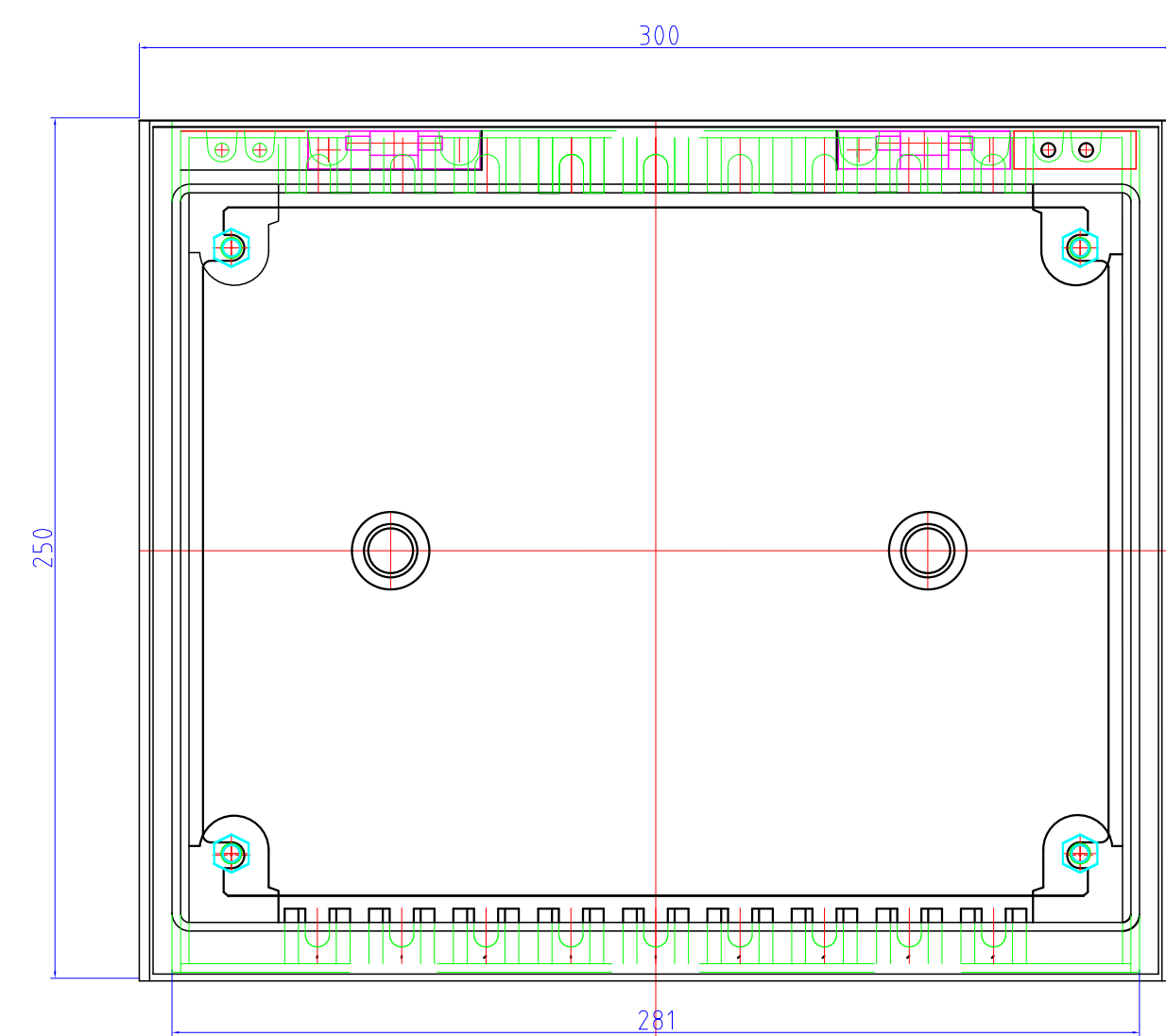
VISTA SUPERIOR
