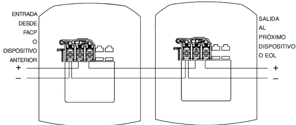
FIGURA 1. CABLEADO DE PRODUCTOS DE 2 CABLES:
