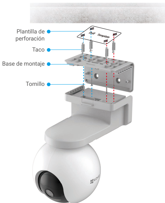
Figura 1. Montaje en techo
