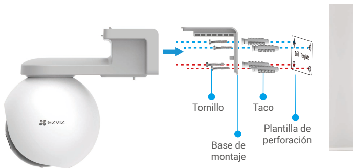
Figura 2. Montaje en pared
