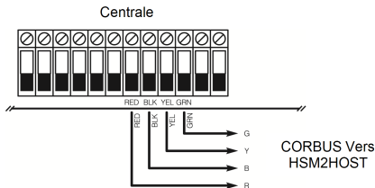
Figure : 1 Schéma de câblage
