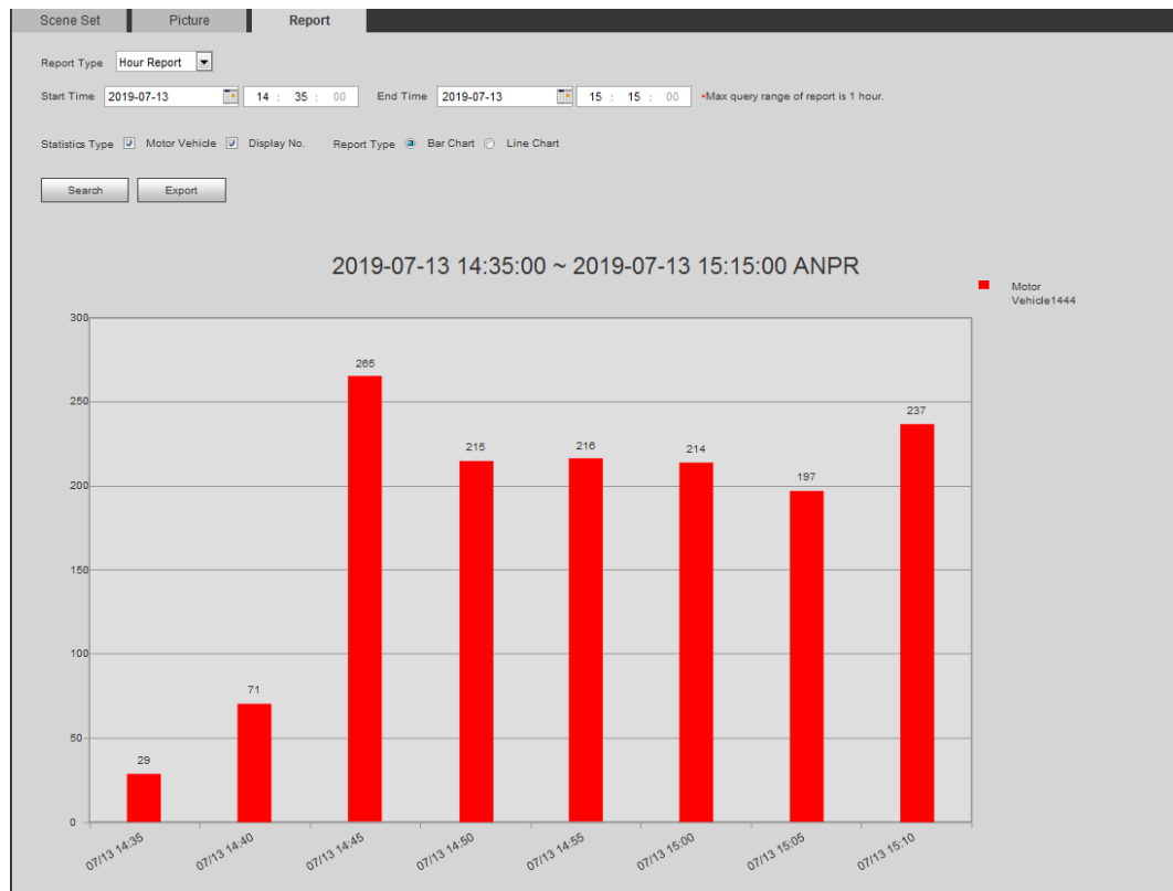
Figura 5-68 Resultados estadísticos
