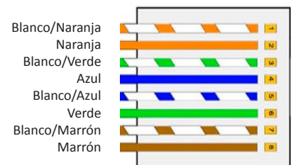
TIA-T568B
