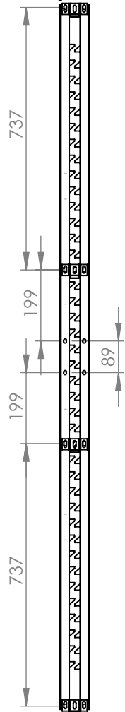
Vista posterior
