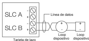
Cableado clase B
