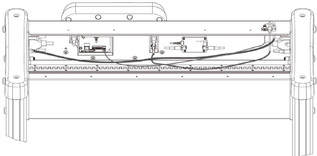
Figura 3-5 Conecte los cables de la cámara
