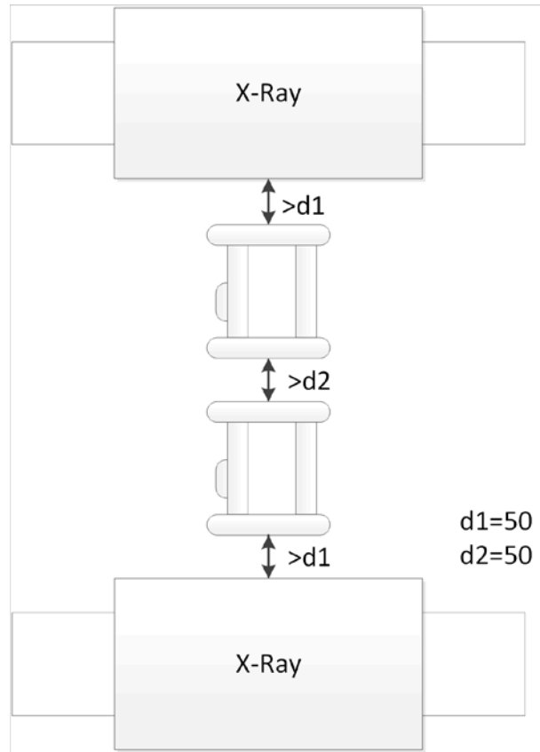
Figura 3-8 Instalación en el sitio de múltiples detectores de paso
