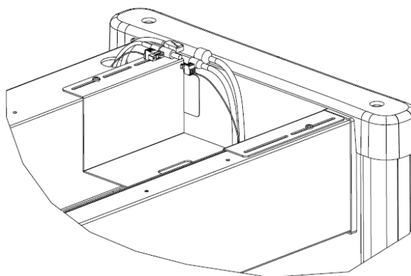
Figura 3-7 Conecte los cables de la cámara
