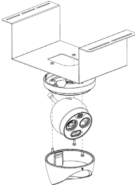
Figura 3-4 Montaje de la cámara
