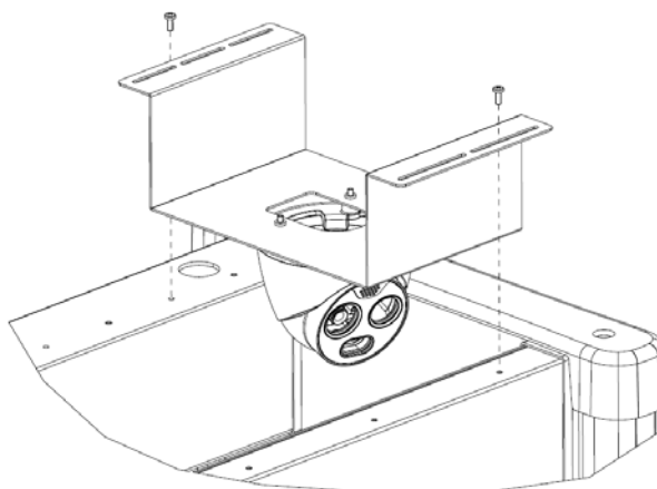
Figura 3-6 Coloque y fije la cámara
