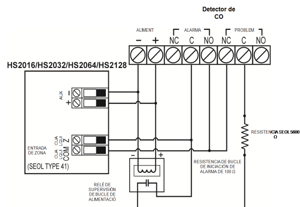
Figura 2-17 Cableado del detector de CO
