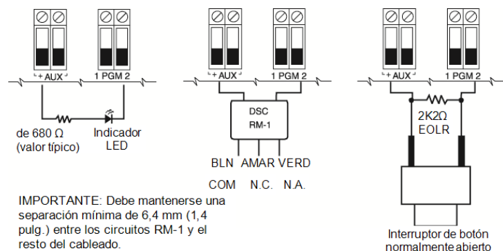
Figura 2-12 Salida LED con resistencia limitadora de corriente y salida opcional de controlador de relé.
