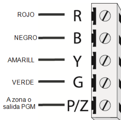
Figura 2-8 Terminales P/Z del teclado
