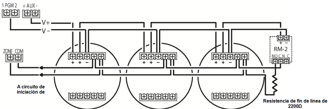
Figura 2-15 Cableado del detector de humo
