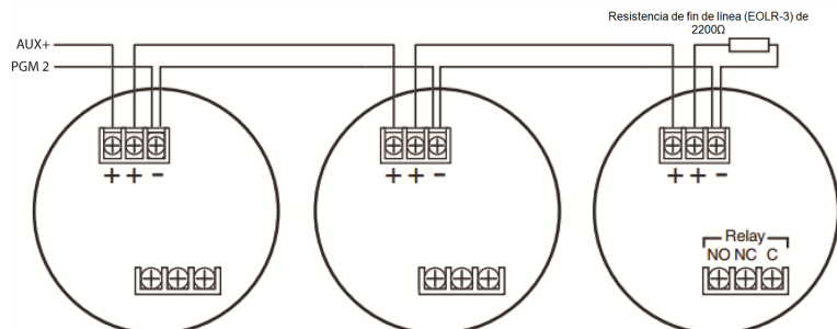
Figura 2-16 Cableado de detector de humos de dos hilos
