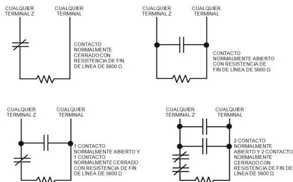
Figura 2-10 Cableado de SEOL
