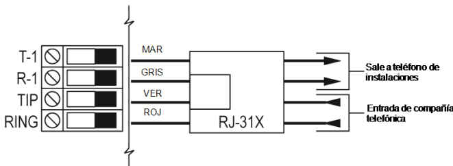
Figura 2-14 Cableado de línea telefónica
