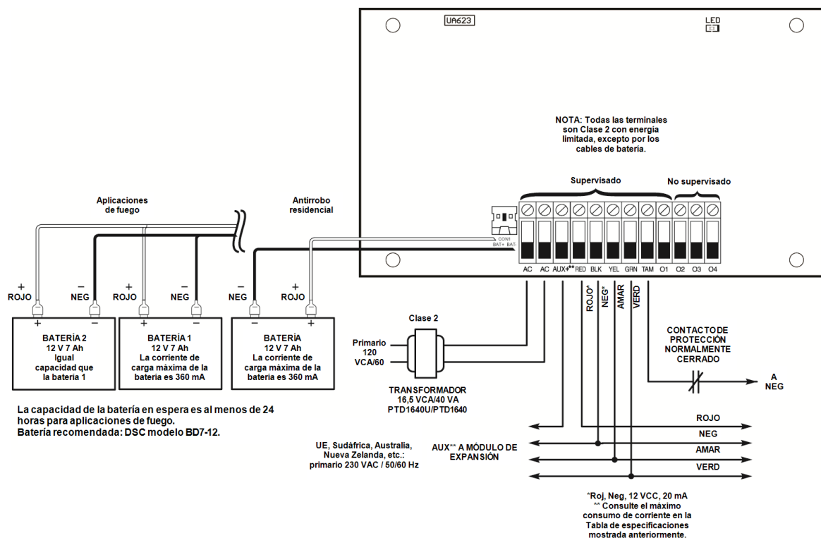
Figura 2-7 Cableado de la fuente de alimentación
