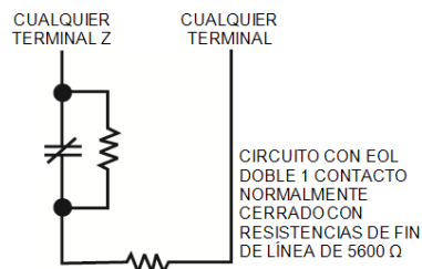
Figura 2-11 Cableado de DEOL
