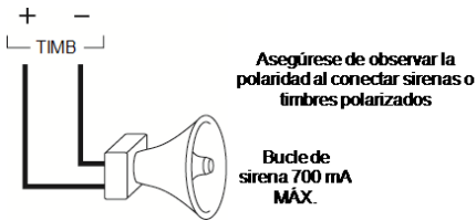
Figura 2-13 Cableado de terminales sirena
