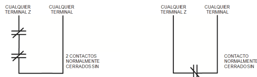
Figura 2-9 Normalmente cerrado
