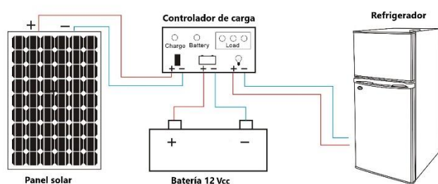
Diagrama de conexión en 12 Vcc
