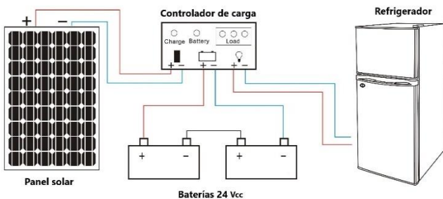
Diagrama de conexión en 24 Vcc
