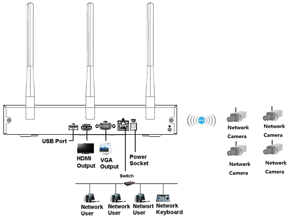
Figura 3-44 Conexión típica
