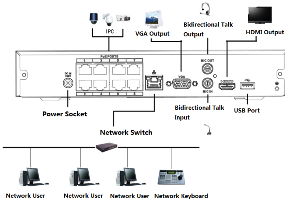
Figura 3-45 Conexión típica
