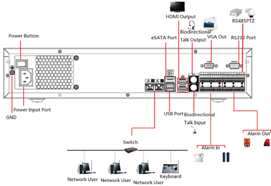
Figura 3-52 Conexión típica
