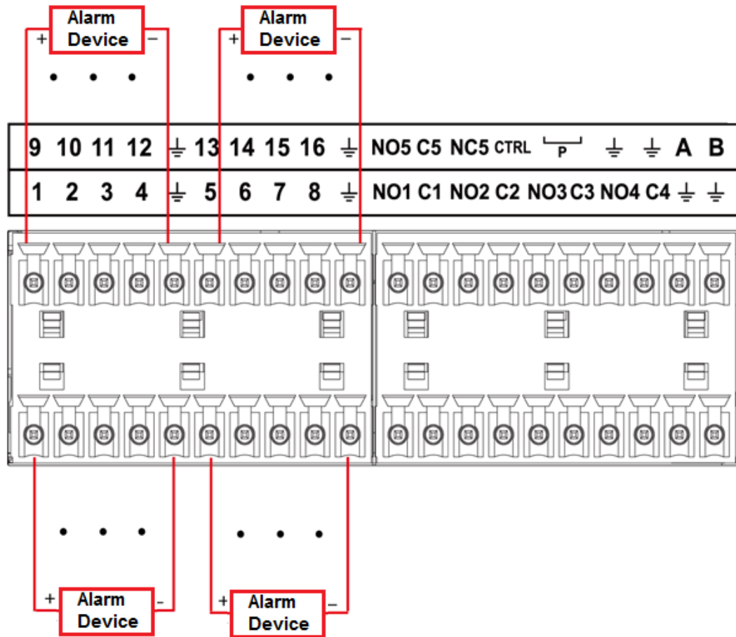
Figura 2-82 Puerto de entrada de alarma
