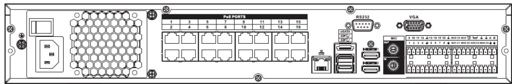
Figura 2-40 Panel trasero
