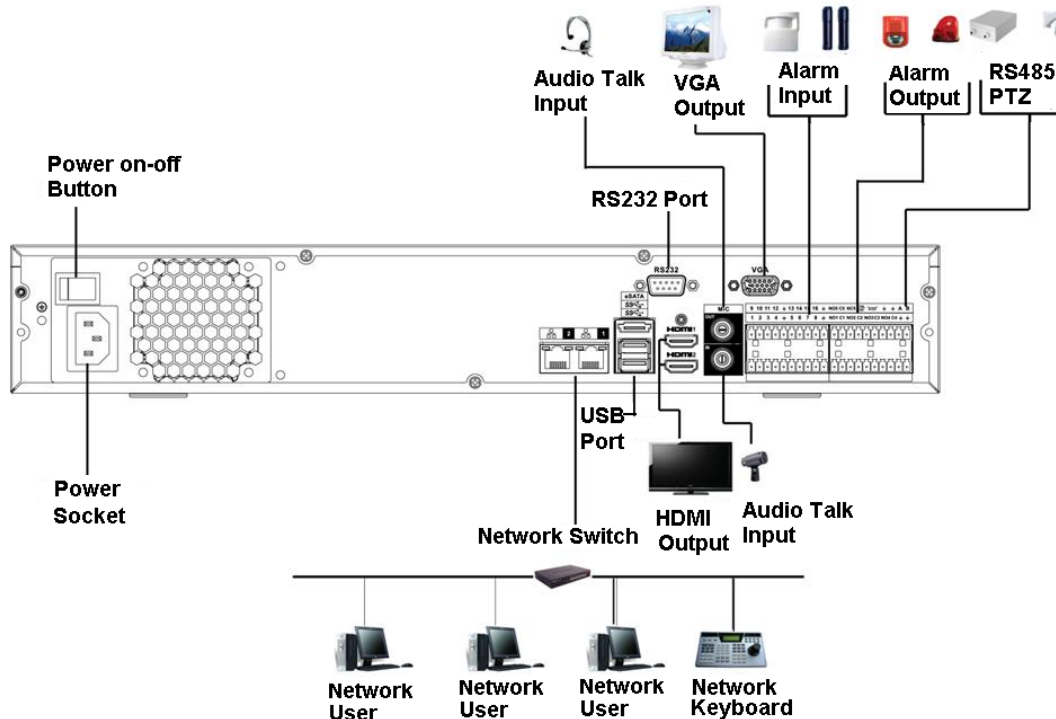
Figura 3-49 Conexión típica
