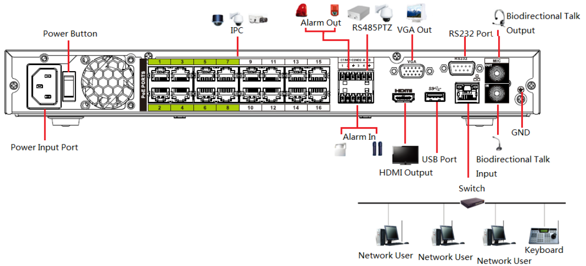
Figura 3-54 Conexión típica
