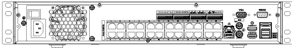
Figura 2-41 Panel trasero
