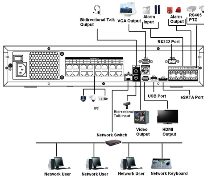
Figura 3-51 Conexión típica
