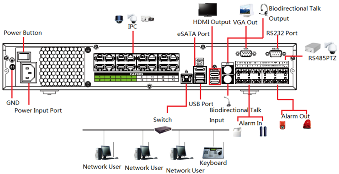
Figura 3-53 Conexión típica
