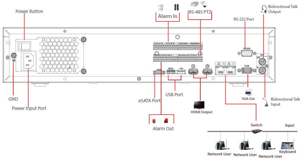
Figura 3-56 Conexión típica
