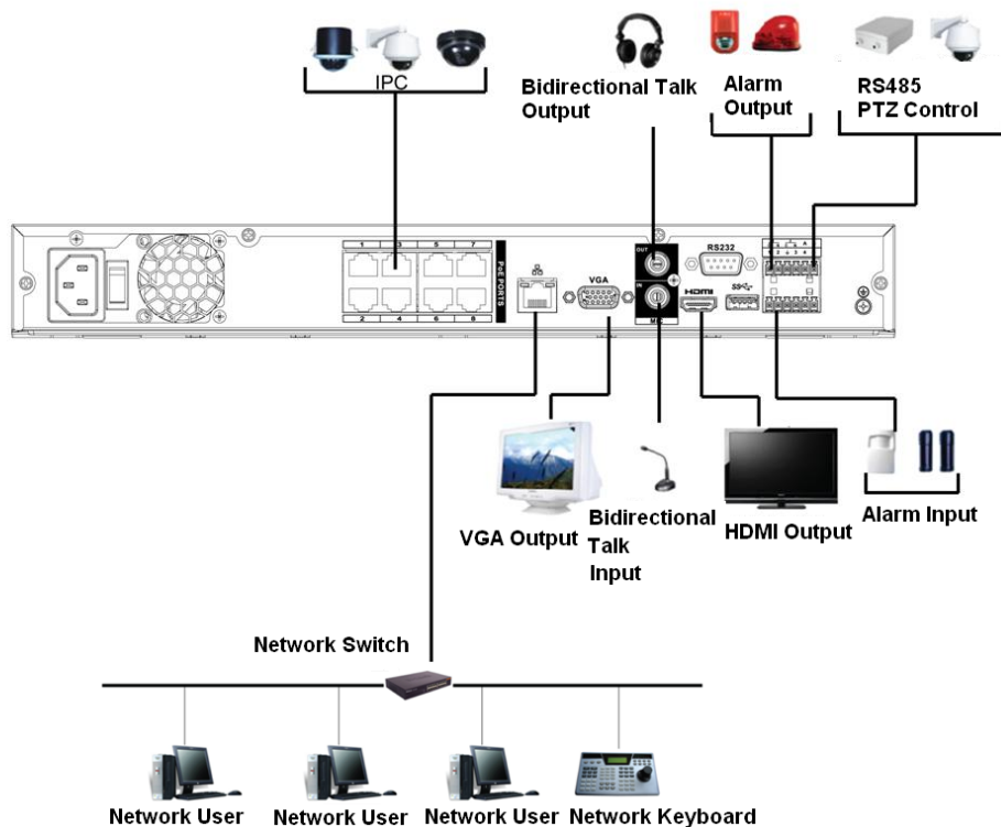
Figura 3-47 Conexión típica
