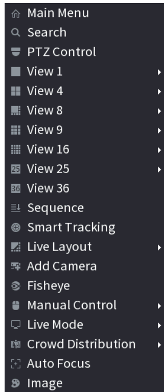
Figura 5-21 Menú contextual (2)
