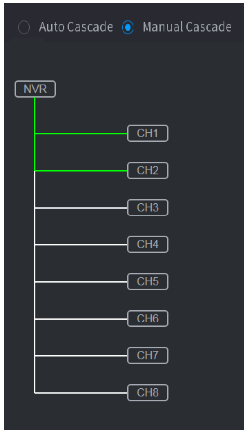
Figura 5-189 Cascada manual
