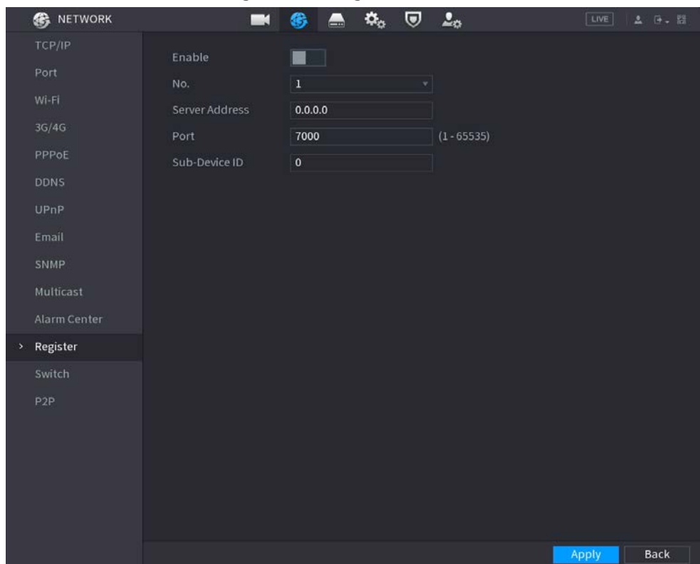
Figura 5-198 Registro
