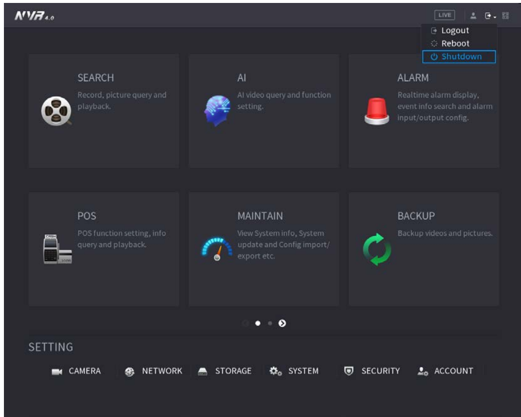
Figura 5-287 Apagado (1)
