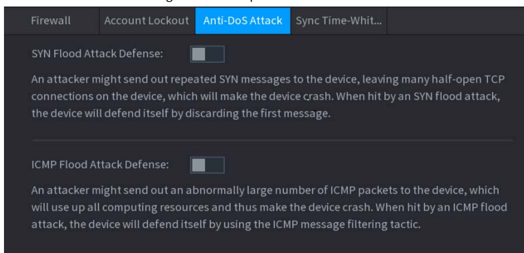
Figura 5-243 Ataque Anti-Dos
