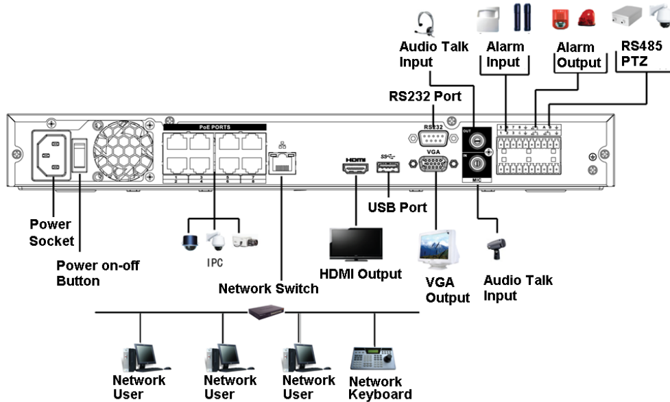
Figura 3-48 Conexión típica
