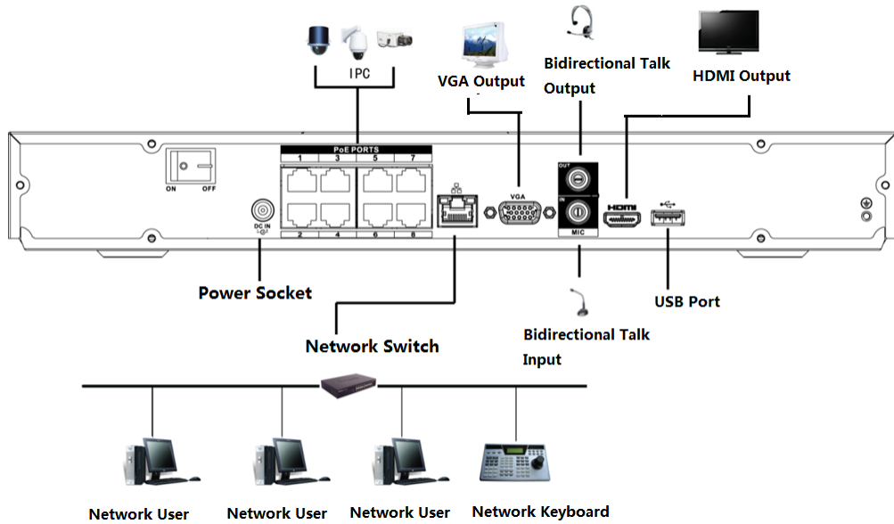
Figura 3-46 Conexión típica
