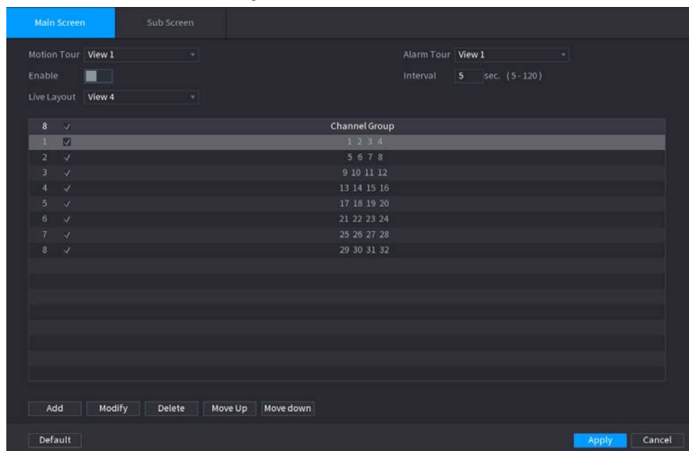
Figura 5-258 Recorrido
