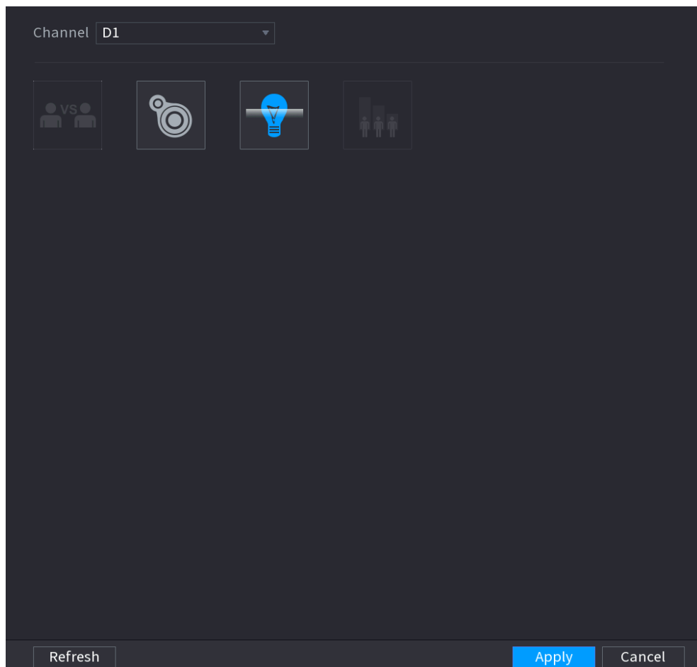
Figura 5-82 Plan inteligente
