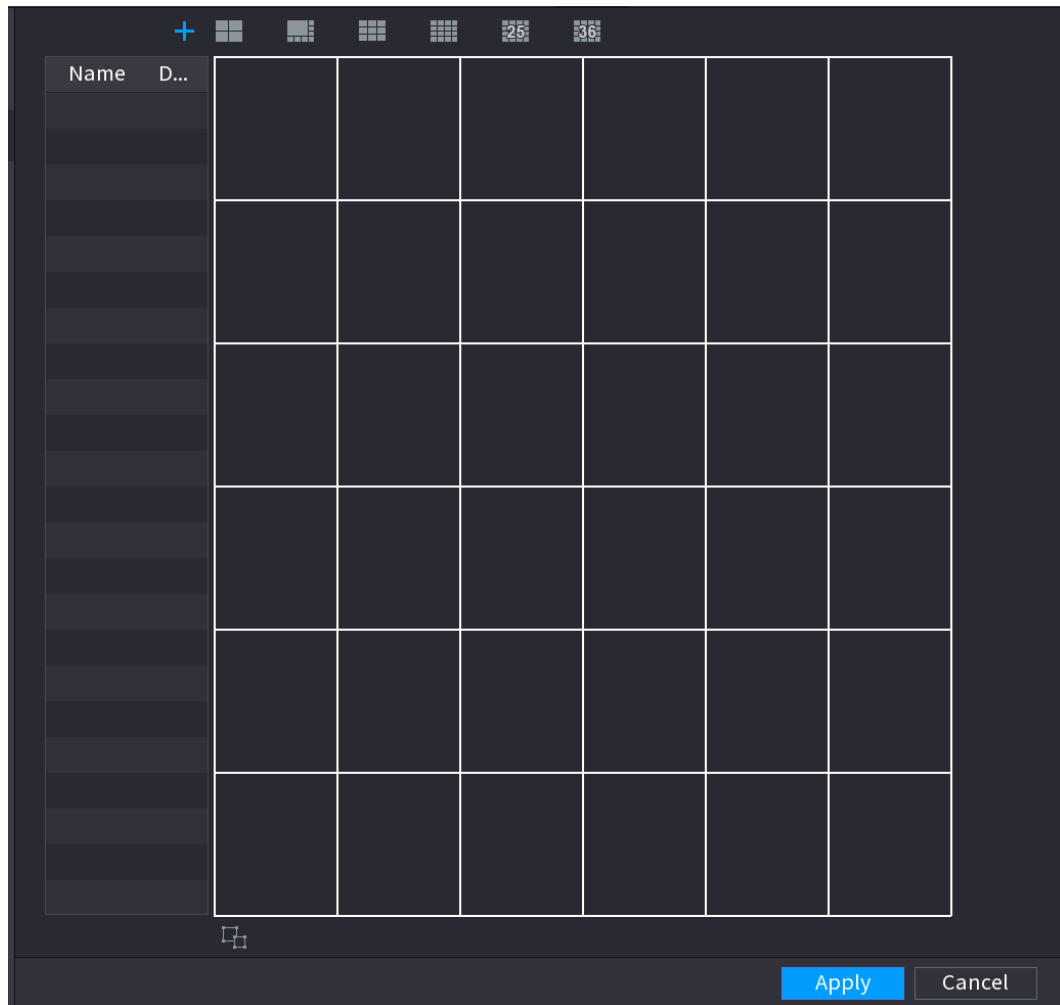
Figura 5-259 División personalizada
