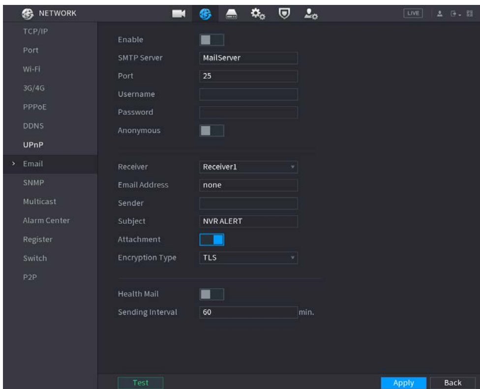
Figura 5-194 Correo electrónico
