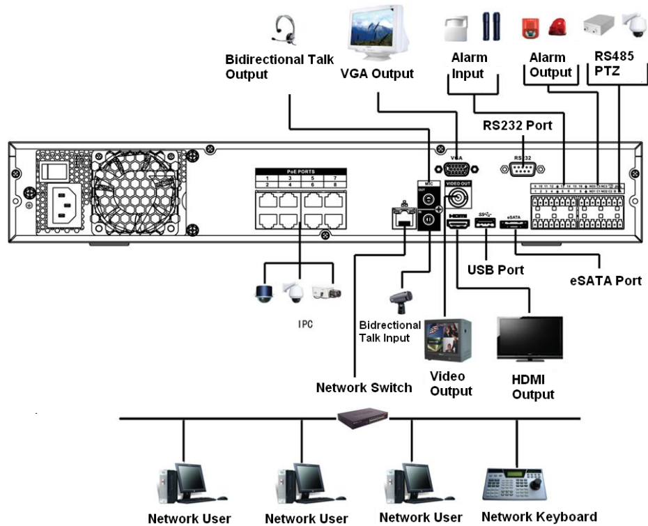
Figura 3-50 Conexión típica
