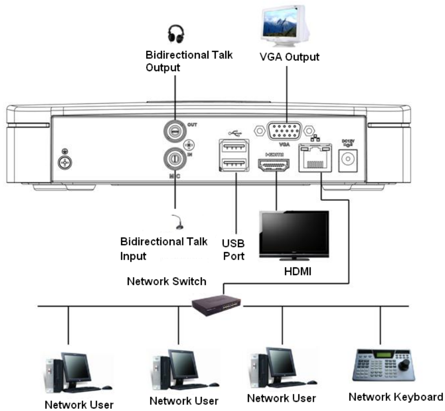
Figura 3-43 Conexión típica
