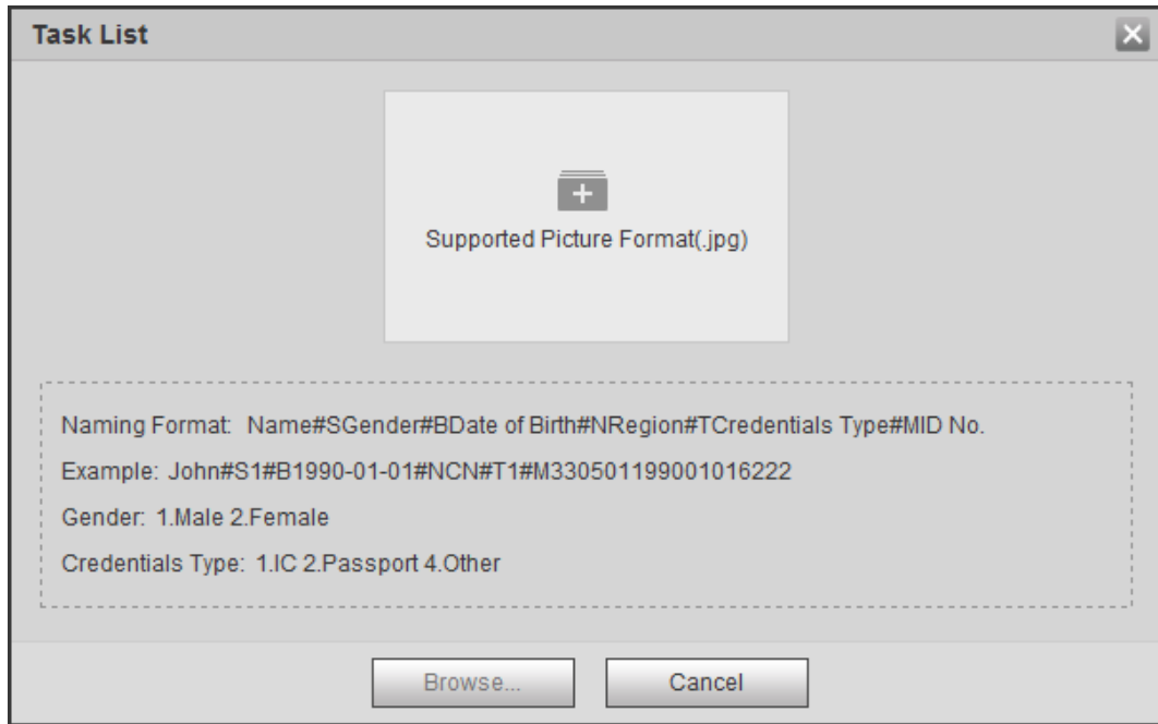
Figura 5-48 Agregar lote
