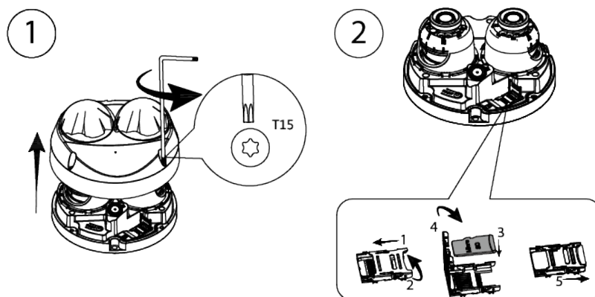
Figura 3-4 Instale la tarjeta SD
