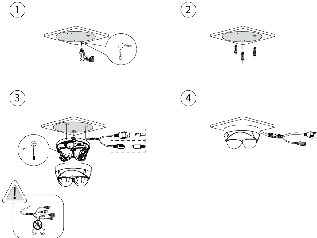
Figura 3-5 Cable pasando por la bandeja portacables lateral
