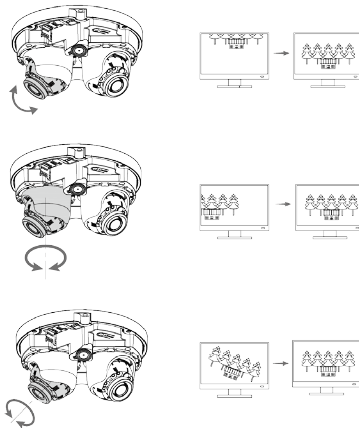
Figura 3-8 Ajuste del ángulo de la lente
