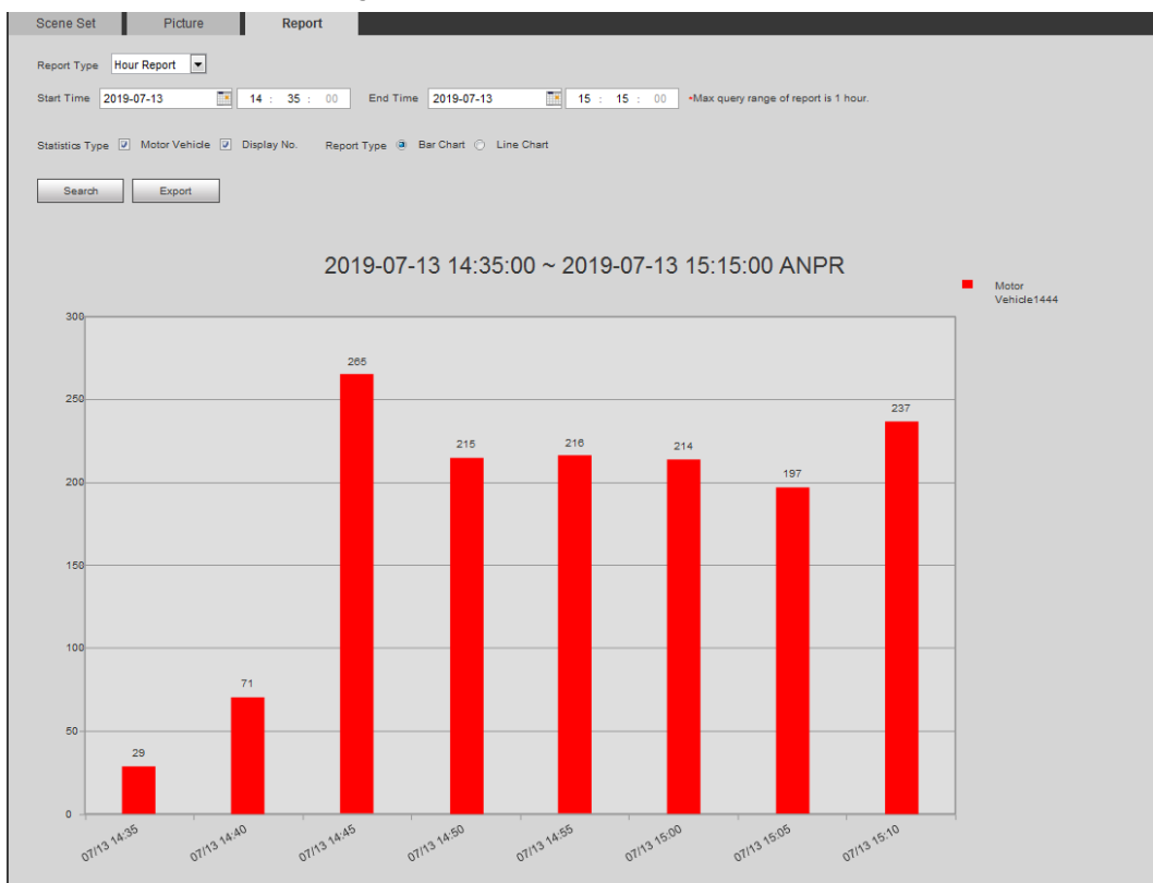
Figura 5-87 Resultados estadísticos
