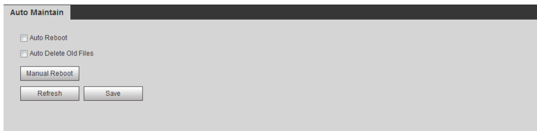
Figura 6-1 Mantenimiento automático
