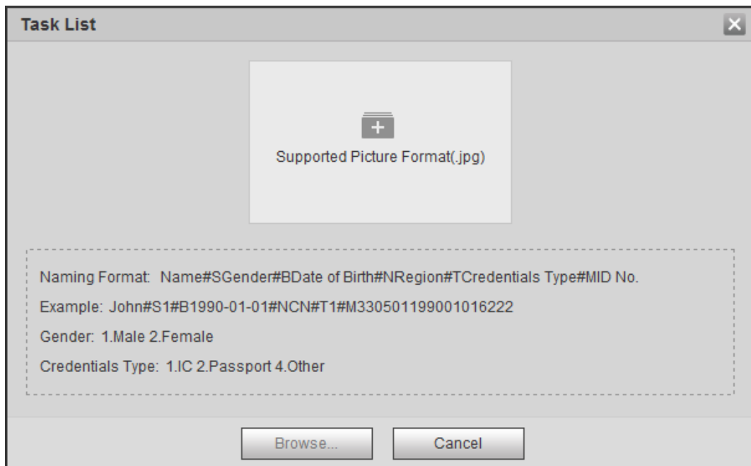
Figura 5-43 Agregar lote
