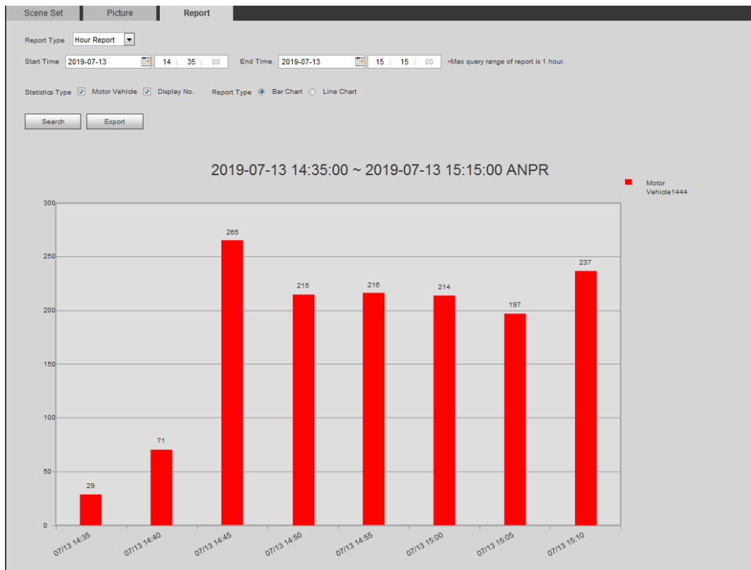
Figura 5-80 Resultados estadísticos
