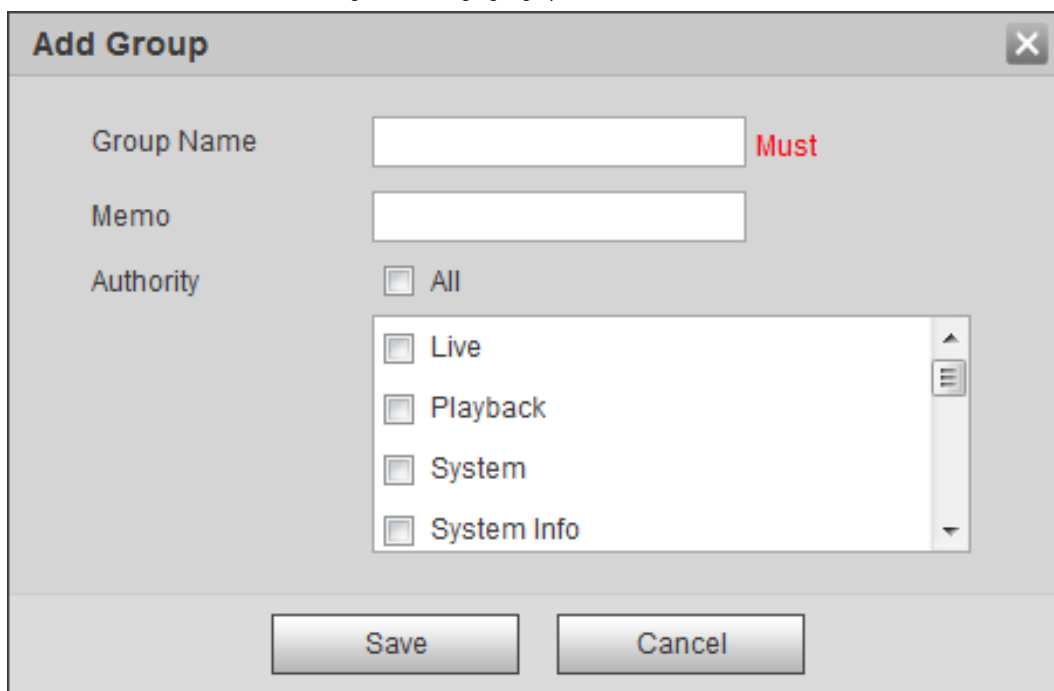
Figura 4-101 Agregar grupo
