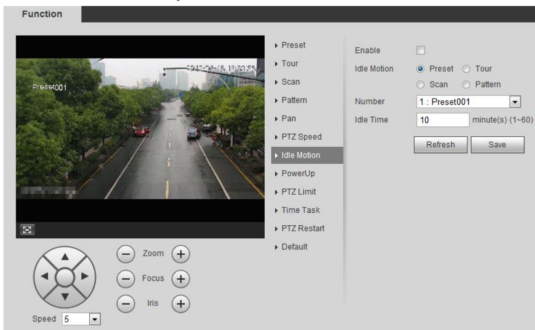
Figura 4-14 Movimiento inactivo
