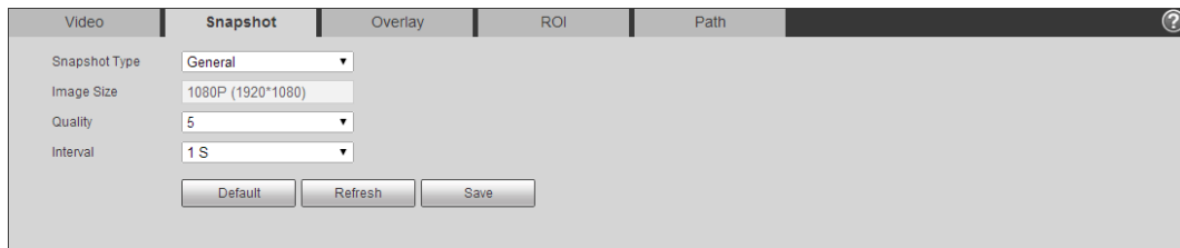
Figura 4-51 Instantánea
