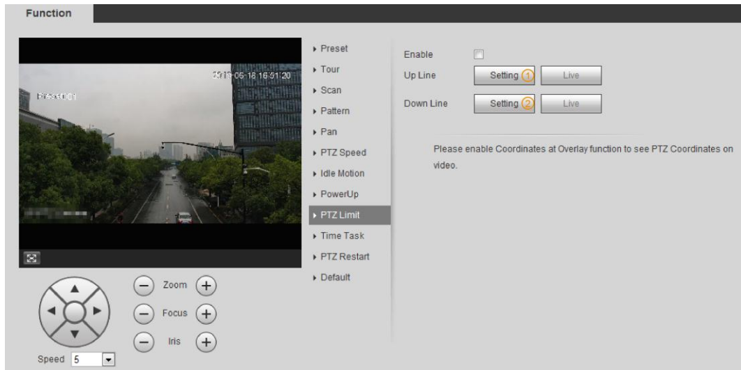
Figura 4-16 Límite PTZ
