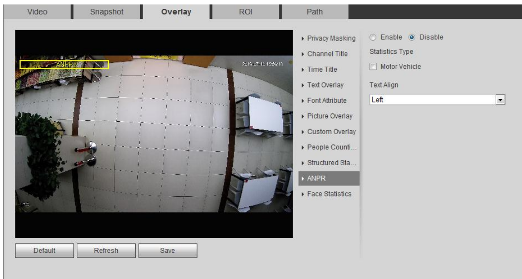
Figura 4-64 ANPR
