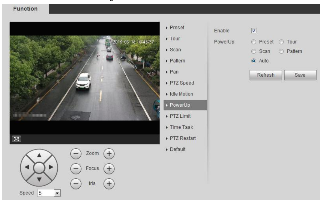
Figura 4-15 Encendido
