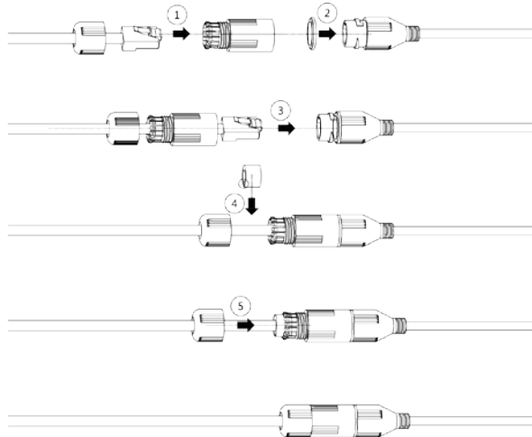
Figura 3-8 Instale el conector a prueba de agua
