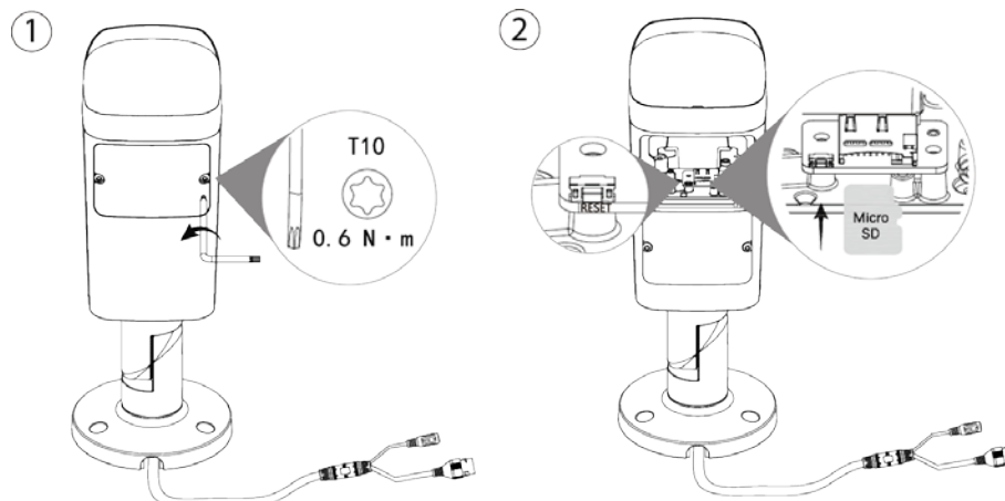
Figura 3-5 Instale la tarjeta SD
