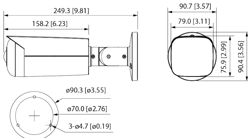
Figura 3-3 Dimensiones: Modelo B (mm [pulgadas])
