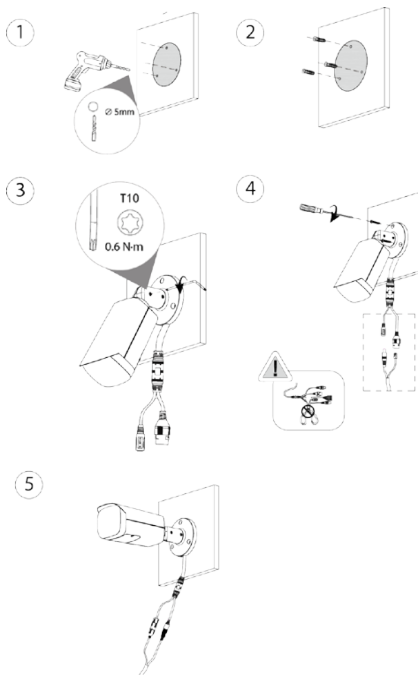
Figura 3-7 Cable que atraviesa la superficie de montaje
