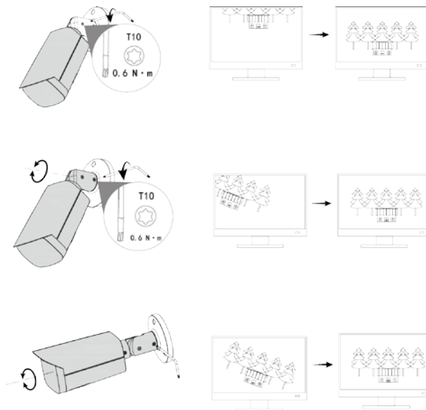
Figura 3-9 Ajuste del ángulo de la lente
