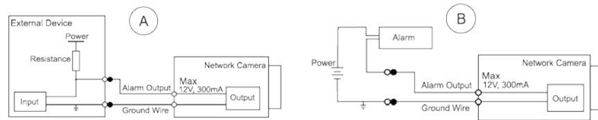
Figura 1-3 Salida de alarma
