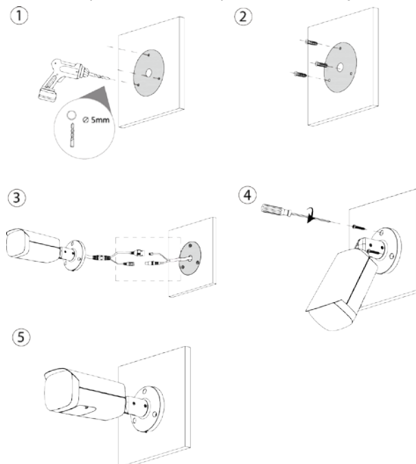
Figura 3-7 Cable que atraviesa la superficie de montaje
