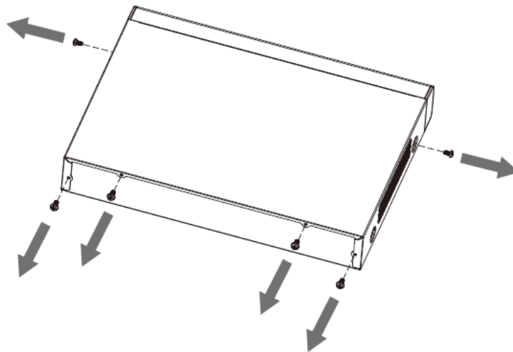
Figure 2-24 Retire los tornillos
