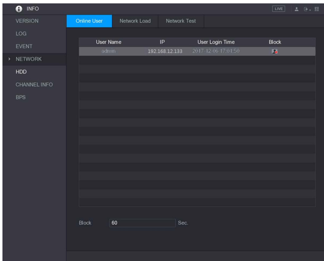
Figure 5-354 Usuario en línea
