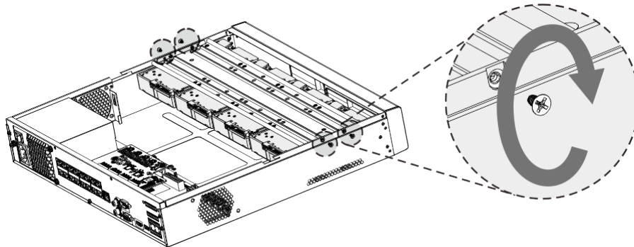
Figure 2-21 Apriete los tornillos
