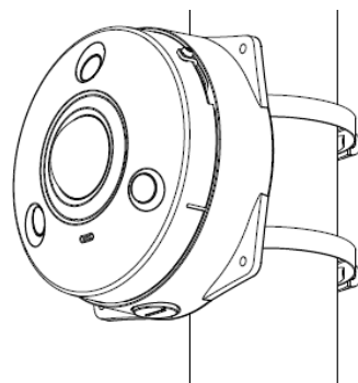
Montaje en poste
