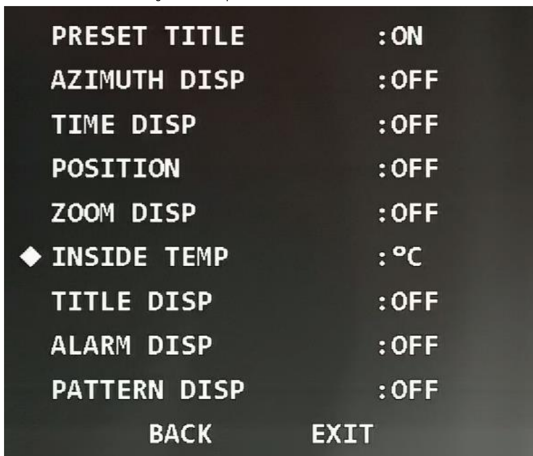
Figura 3-27 Temperatura interior
