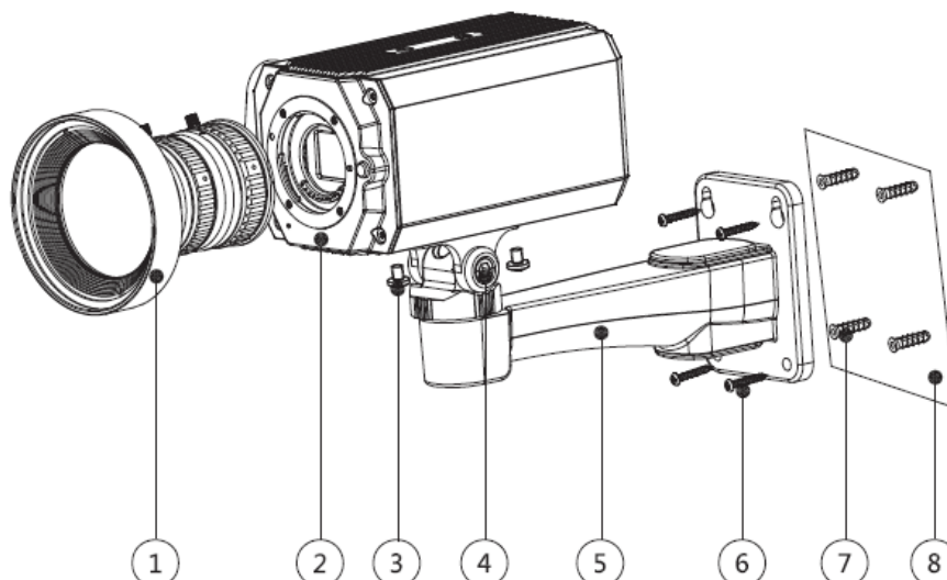
Figura 9-6 Componentes del dispositivo
