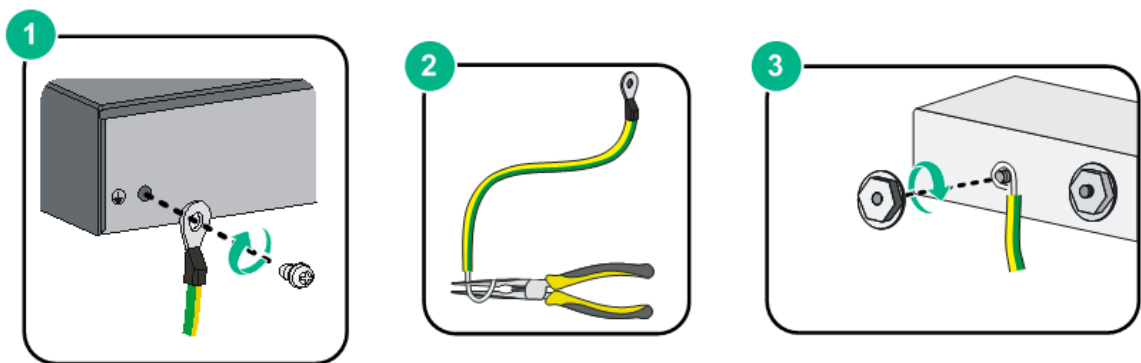
Figura 4-1 Conexión GND
