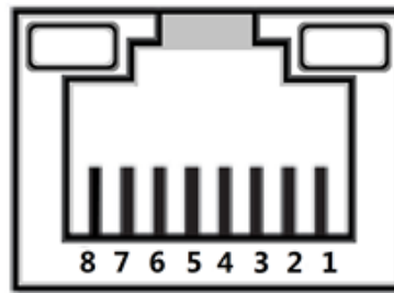
Figura 4-3 Descripción de pines
