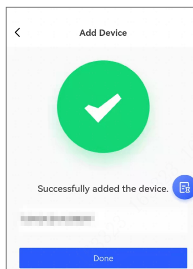
Figura 5-4 Agregar dispositivo
