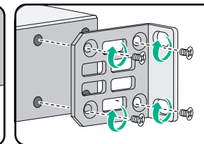
Coloque un soporte de montaje frontal tipo A cerca del lado del módulo de alimentación.
