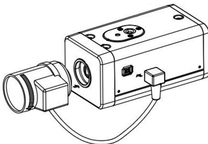
Figure 9-1 Instalación de lentes (1)
