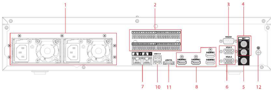
Figura 2-110 Panel trasero (5)
