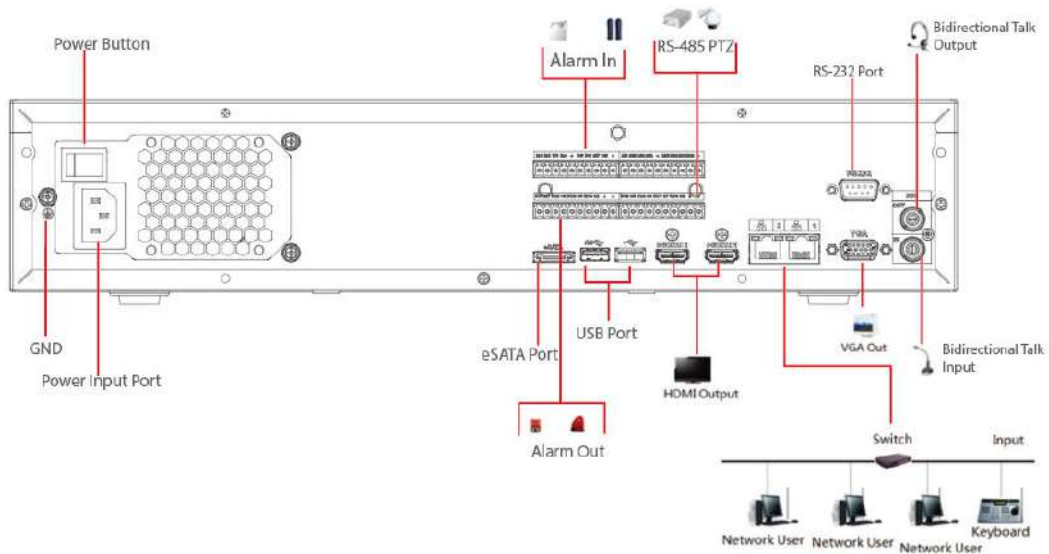
Figura 3-61 Conexión típica
