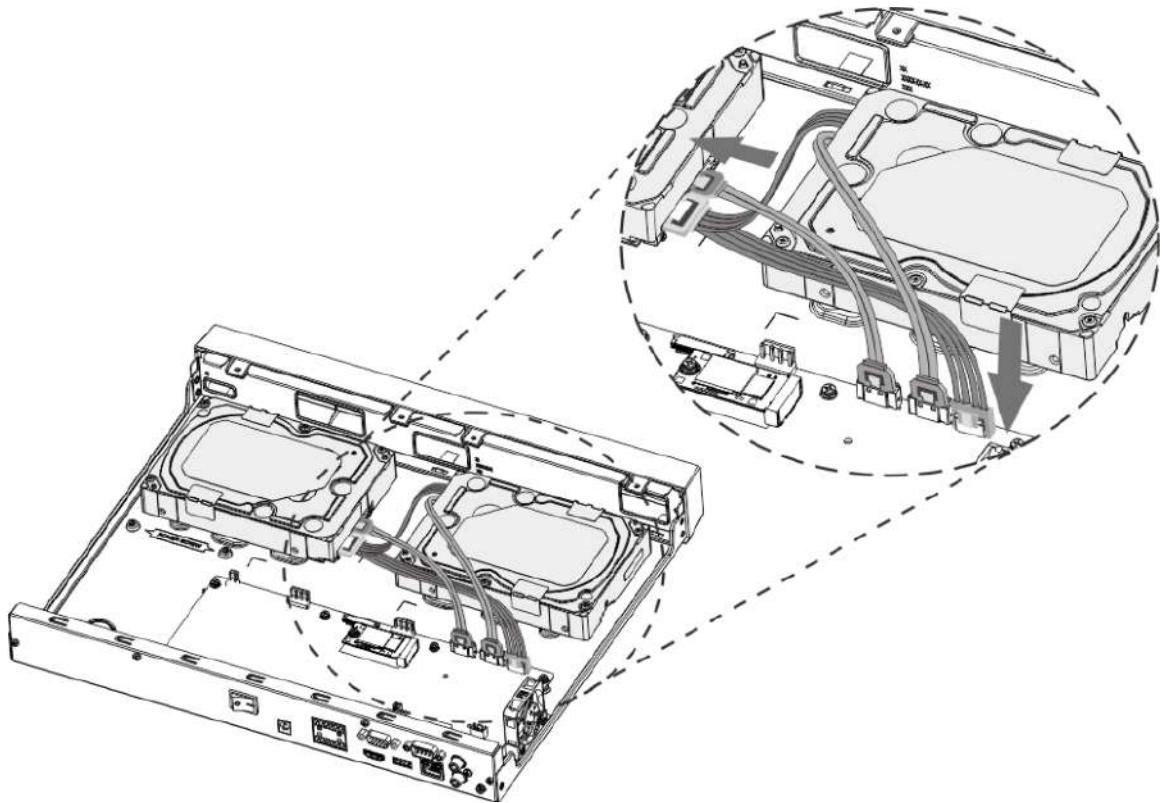
Figura 3-16 Conexión de cables
