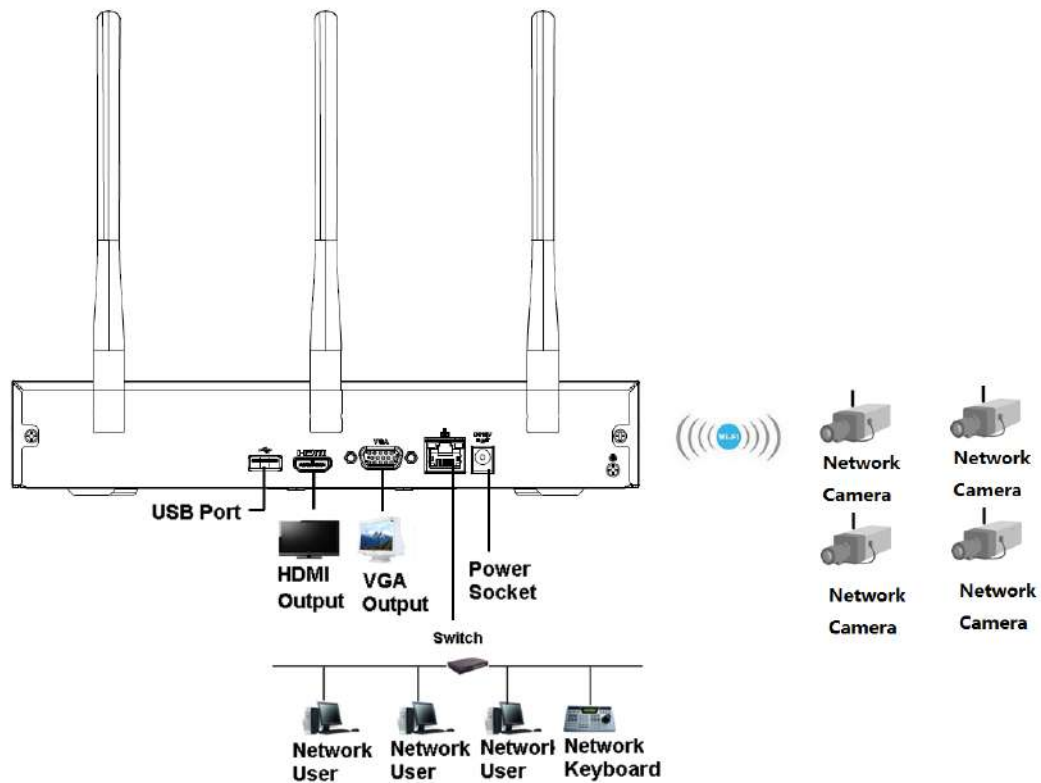
Figura 3-49 Conexión típica
