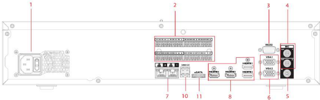
Figura 2-109 Panel trasero (4)
