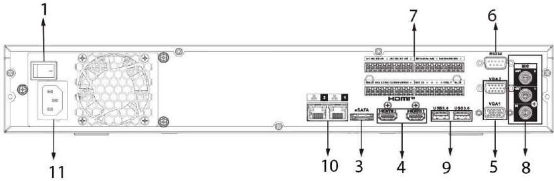
Figura 2-101 Panel trasero (3)
