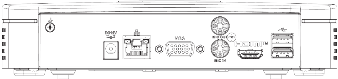
Figura 2-37 Panel trasero
