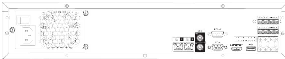
Figura 2-73 Panel trasero
