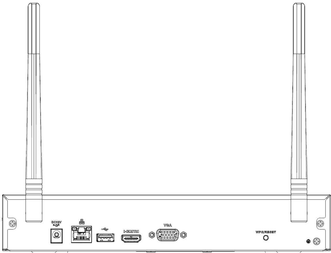
Figura 2-80 Panel trasero
