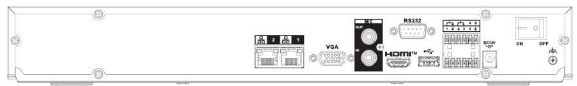
Figura 2-84 Panel trasero (3)
