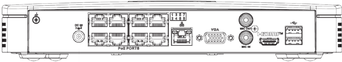
Figura 2-39 Panel trasero
