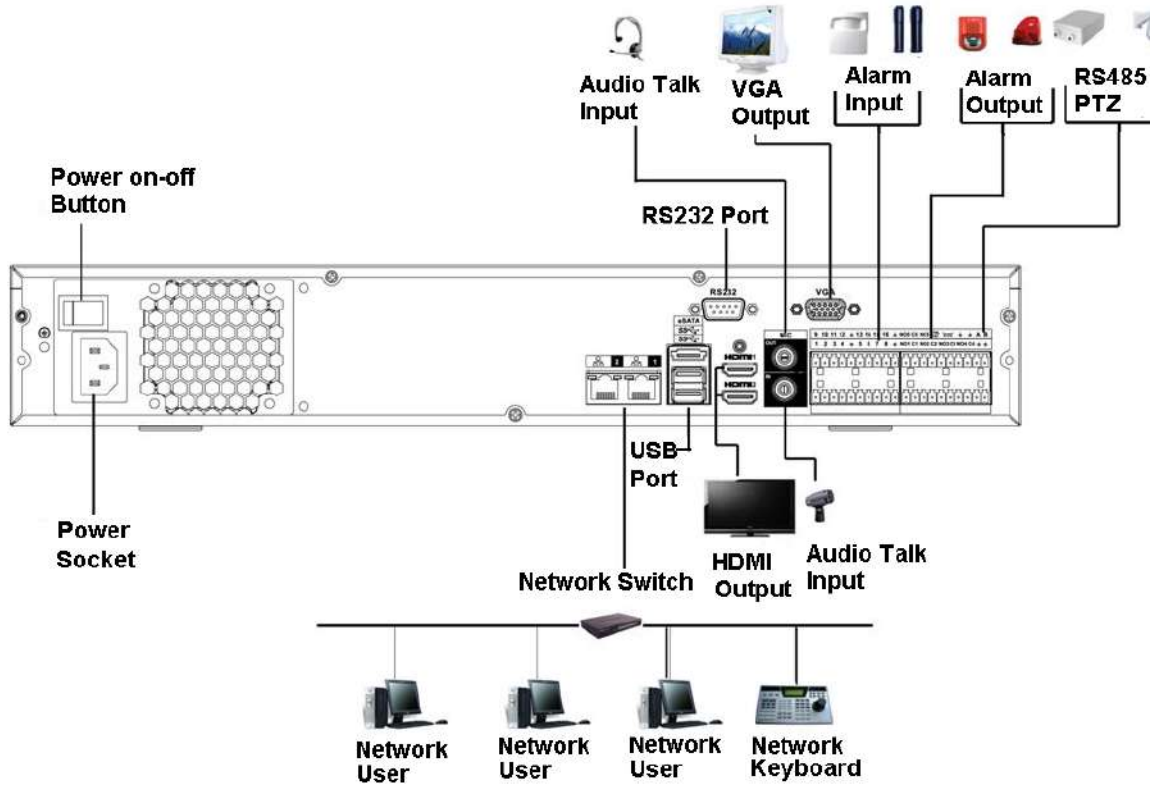
Figura 3-54 Conexión típica
