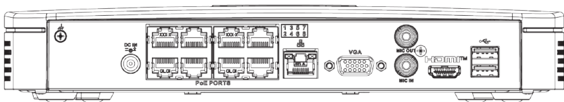
Figura 2-88 Panel trasero
