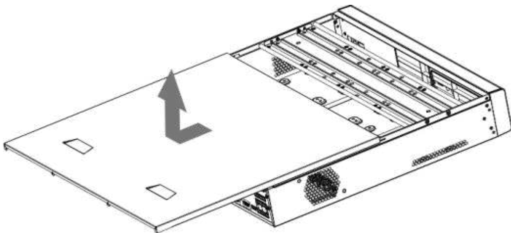
Figura 3-19 Quitar la cubierta
