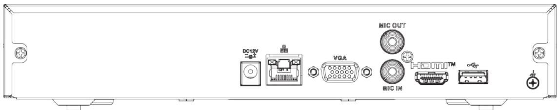
Figura 2-40 Panel trasero
