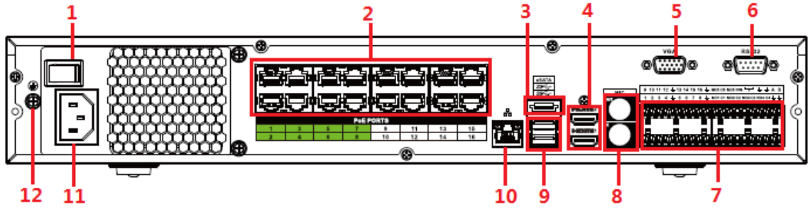
Figura 2-100 Panel trasero (2)
