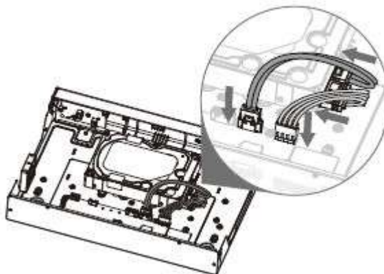
Figura 3-10 Conexión de cables
