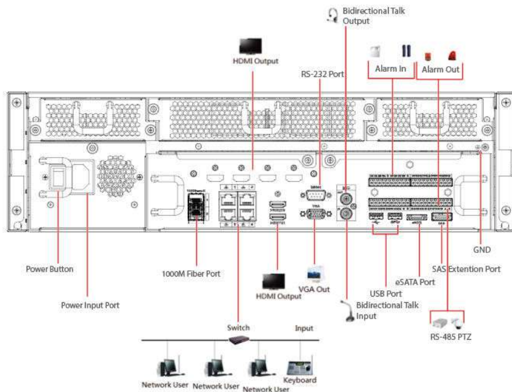
Figura 3-62 Conexión típica
