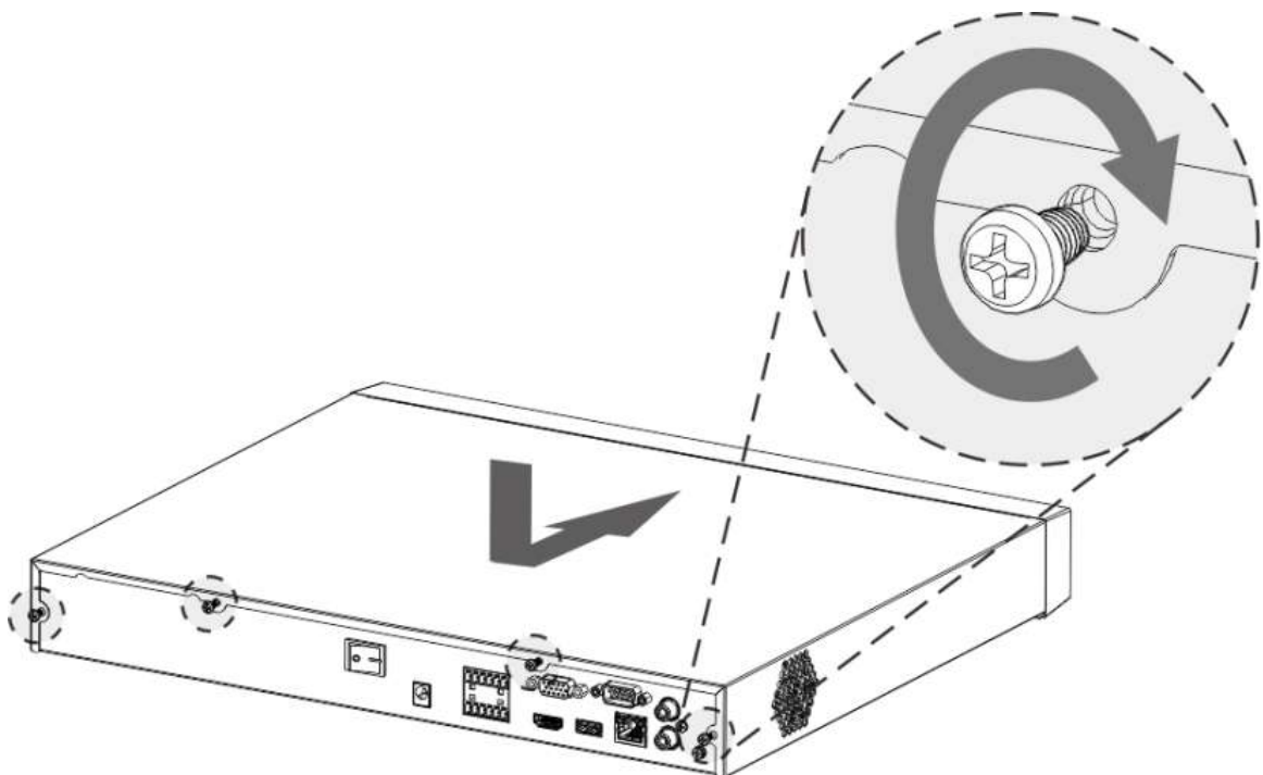
Figura 3-17 Volver a colocar la cubierta
