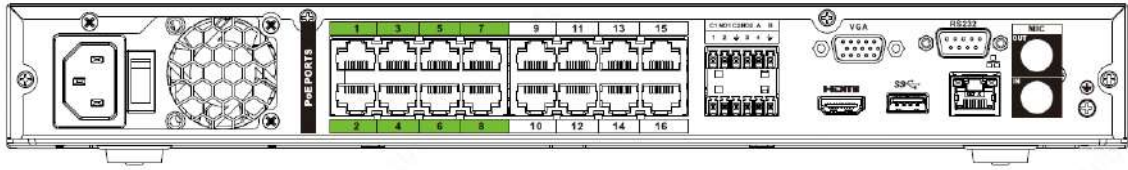
Figura 2-54 Panel trasero
