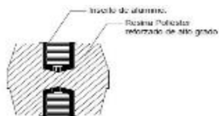
PERSPECTIVAS AISLADOR CORTE TRANSVERSAL
