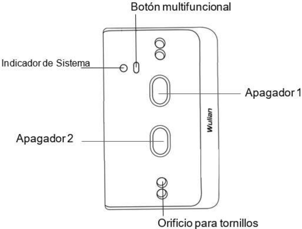
Cuerpo principal
