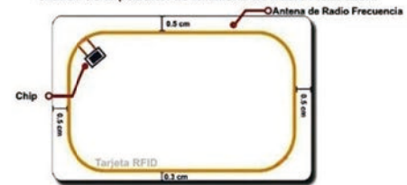
Gráfica de la posición de la antena de Radio Frecuencia
